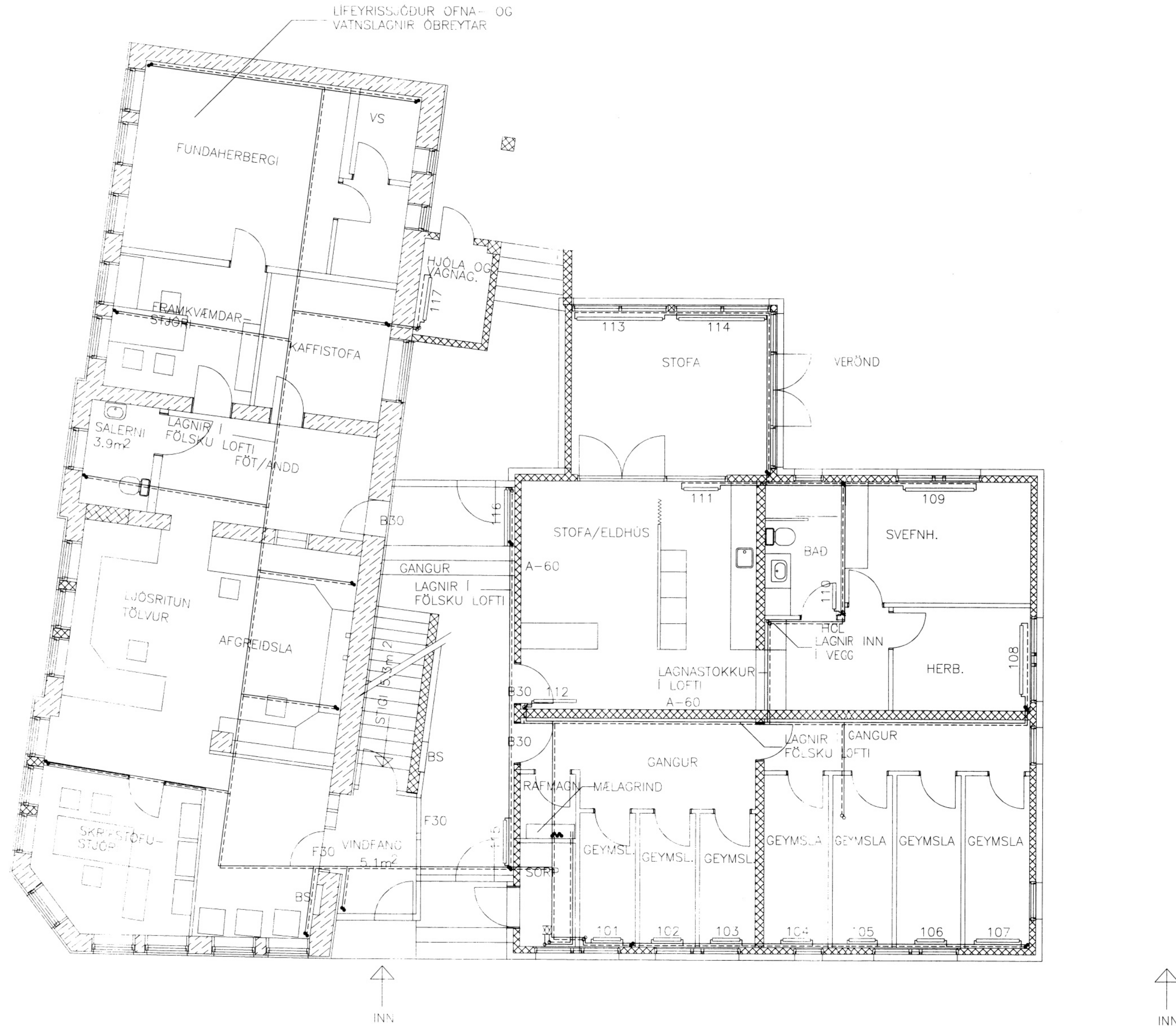
GRUNNMYND 1. HÆÐ
