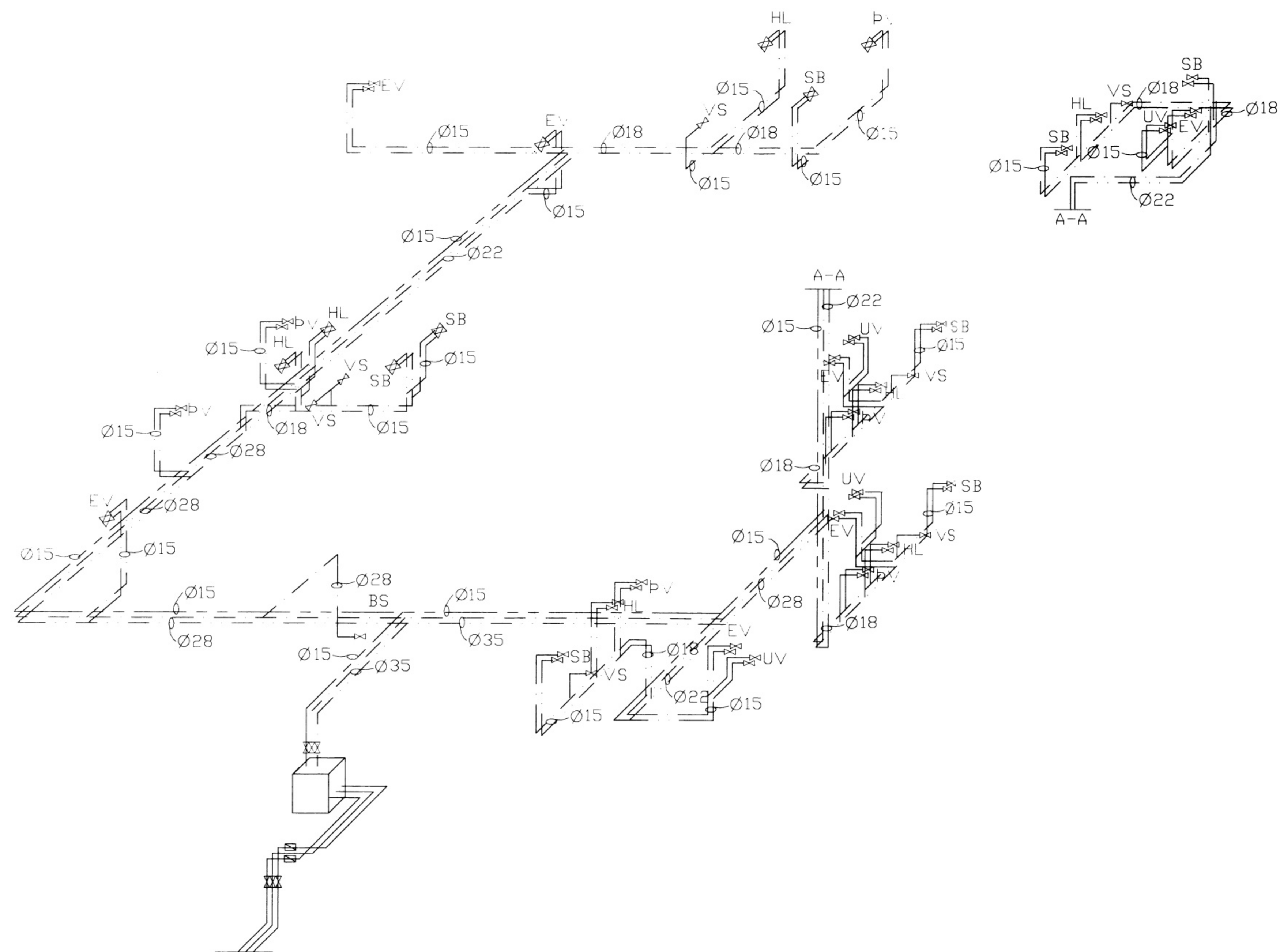
RÚMMYND VATTNSLAGNIR M=1:50
