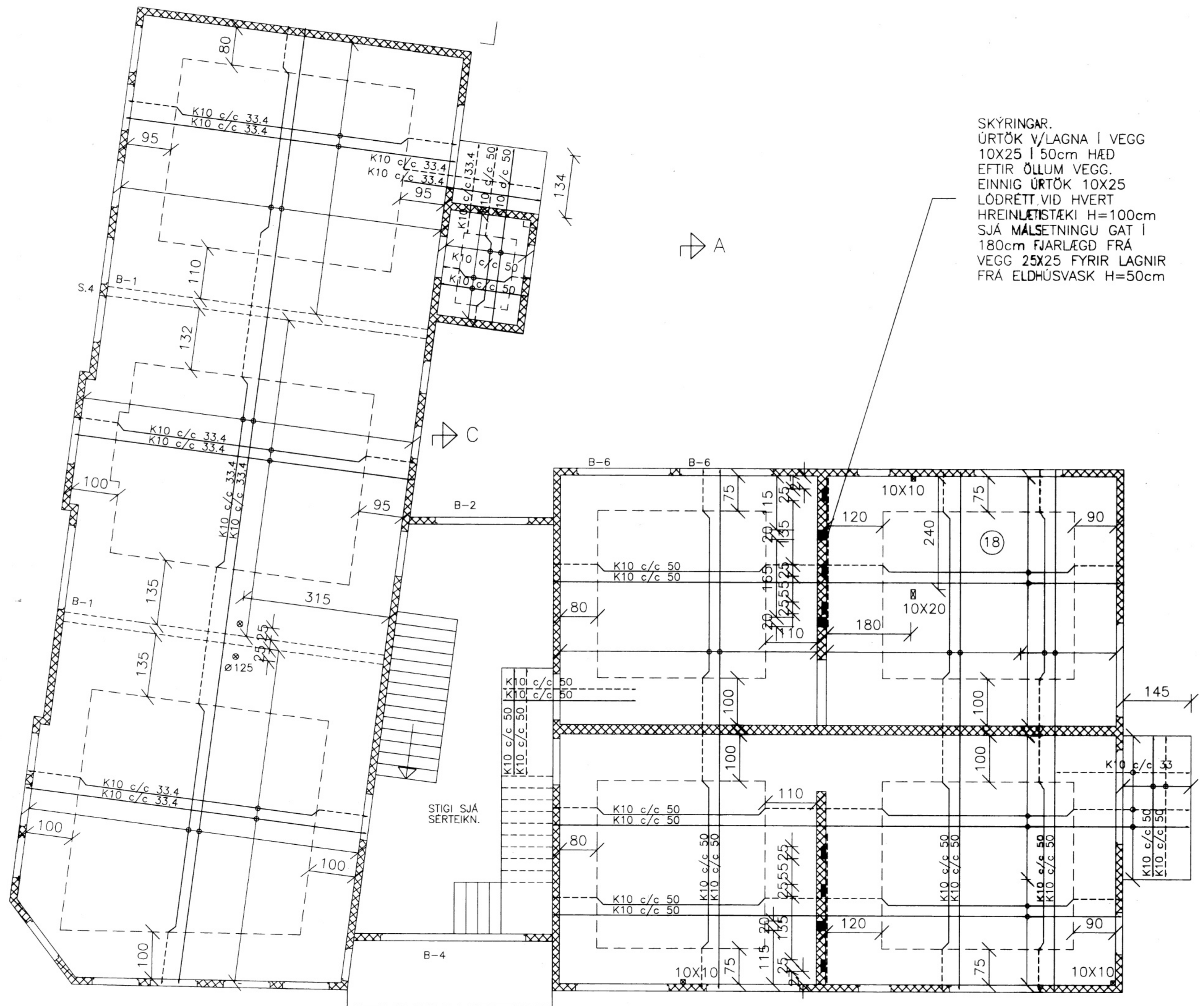
GRUNNMYND PLÖTUR YFIR 2. HÆÐ M=1:50
