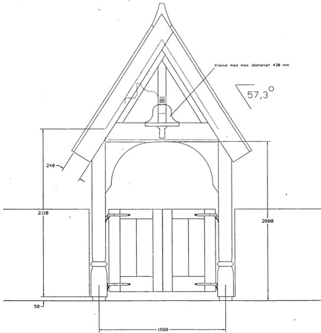
Oppriss ved portal/støpul
