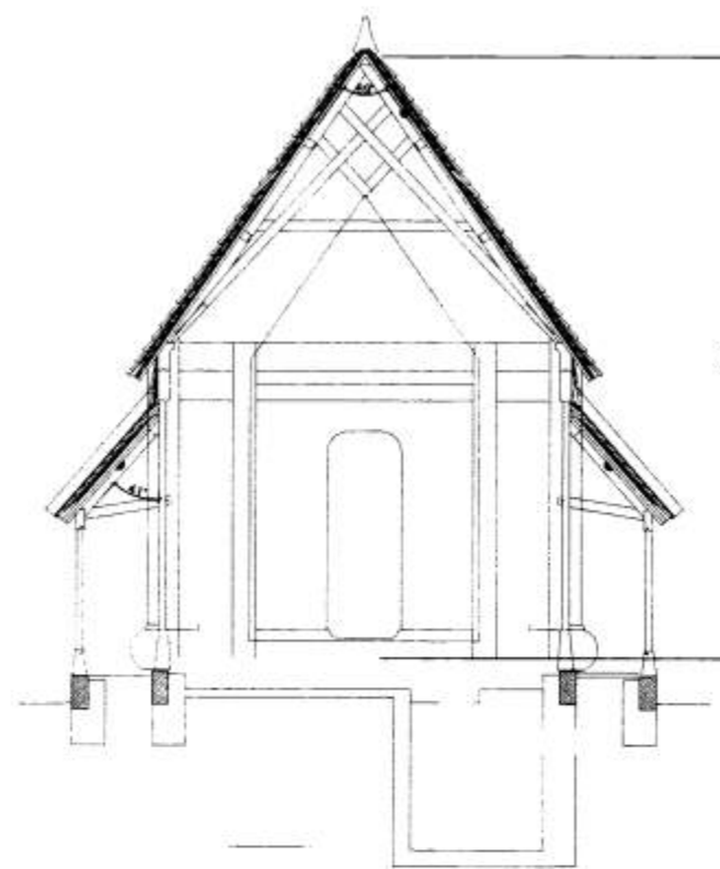
ÞVERSNID
