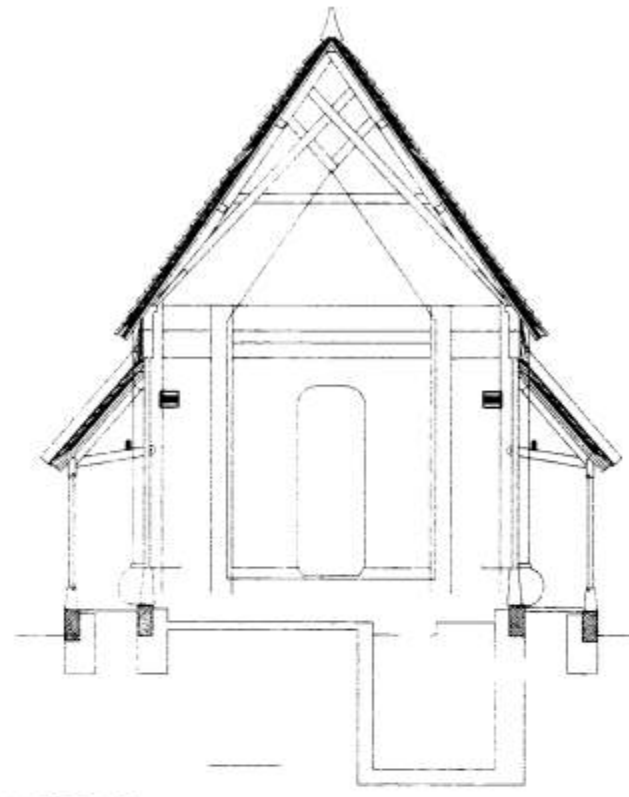
ÞVERSNID
