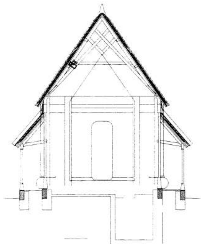
ÞVERSNIÐ
