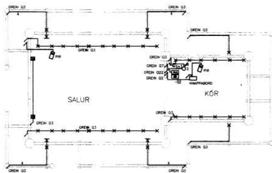
GRUNNMYND
