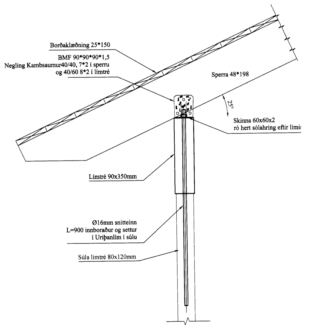
FRÁGANGUR VÍÐ LÍMTRÉ OG SÚLU ÚTI Mkv: 1/10
