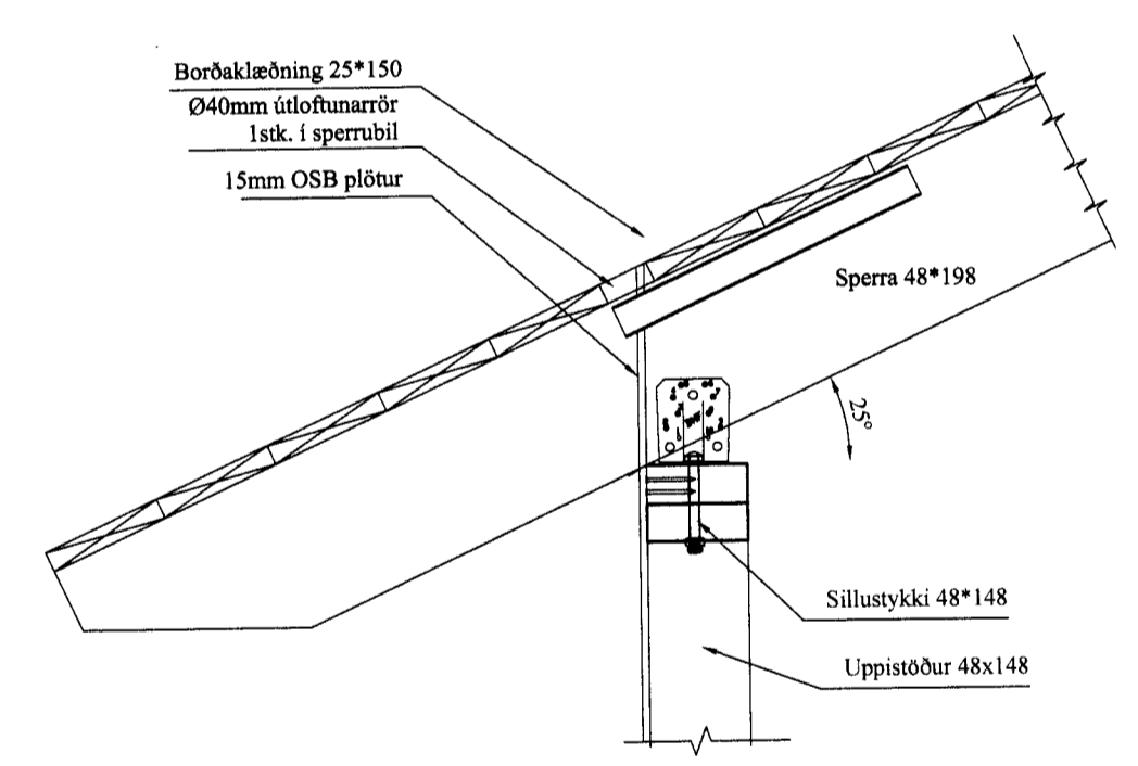
FRÁGANGUR VÍÐ ÞAKKANTA Mkv: 1/10
