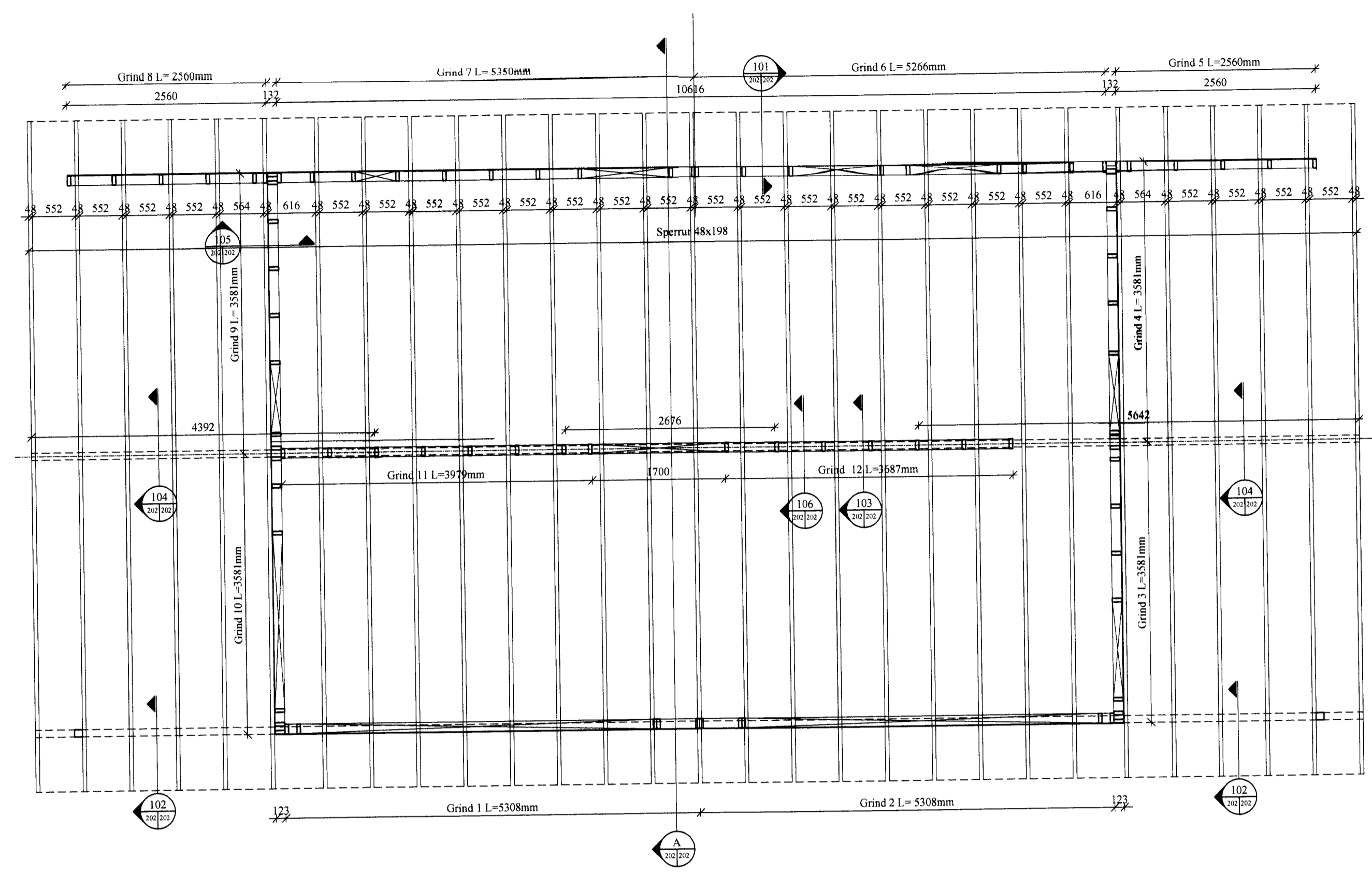
GRUNNMYND VEGGJA, MILLILOFT OG SPERRA NEDRA ÞAKS Mkv: 1/50
