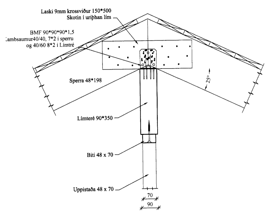
FRÁGANGUR VÍÐ MÆNI Mkv: 1/10
