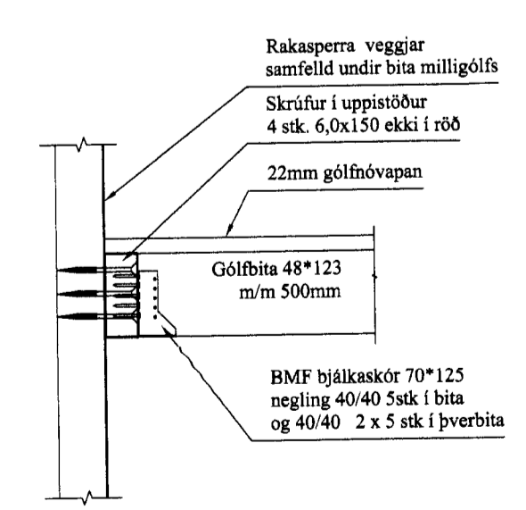
FRÁGANGUR VÍÐ MILLILOFT Mkv: 1/10
