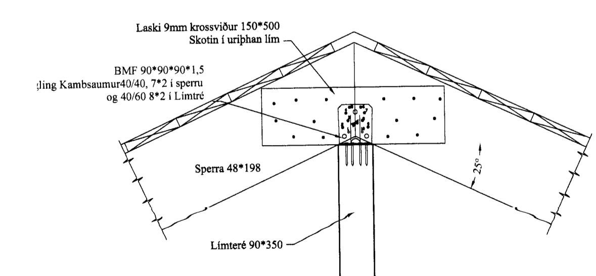
FRÁGANGUR VÍÐ MÆNI ÚTI Mkv: 1/10
