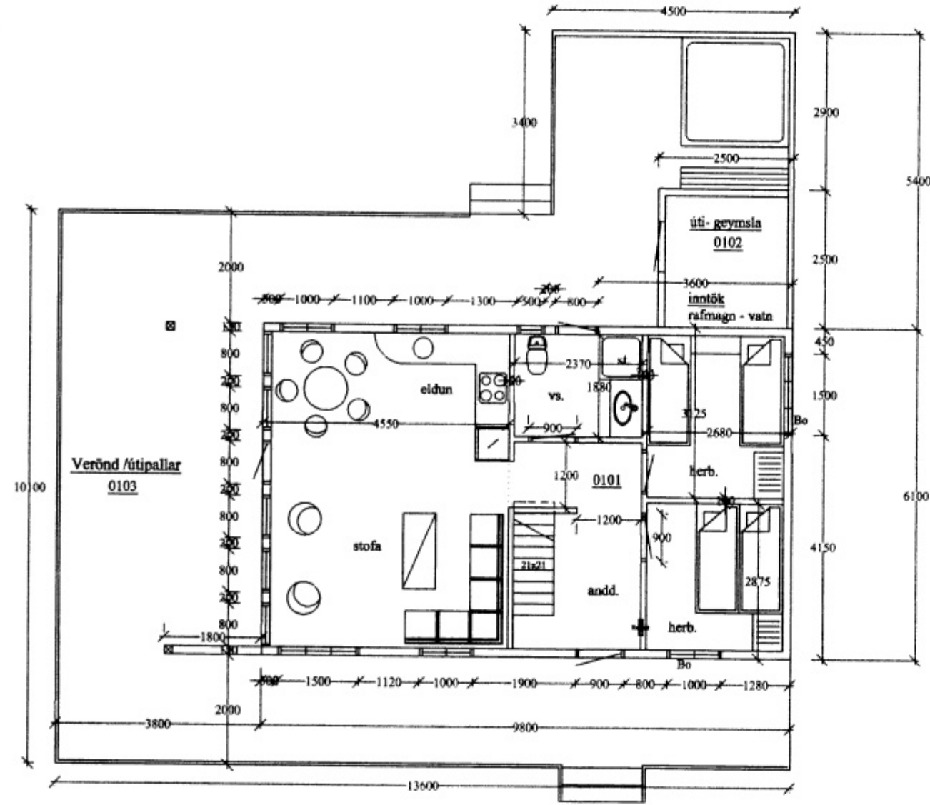
Grunnmynd 1. Hæð M 1:100
