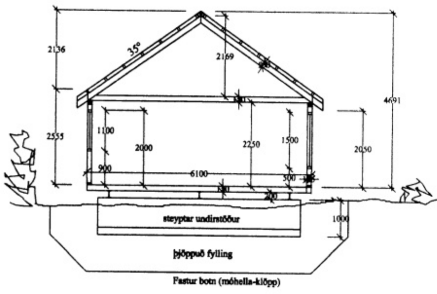
Pversnid M 1:100
