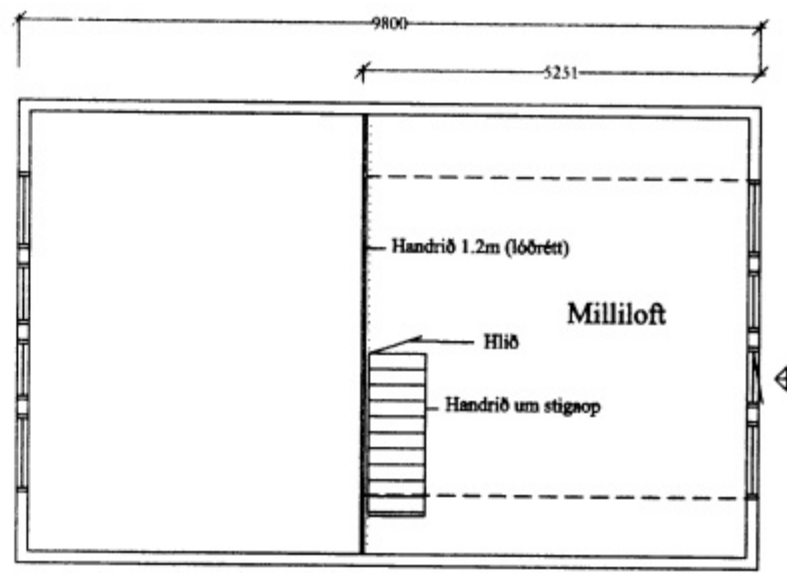
Grunnmynd risloft M 1:100
