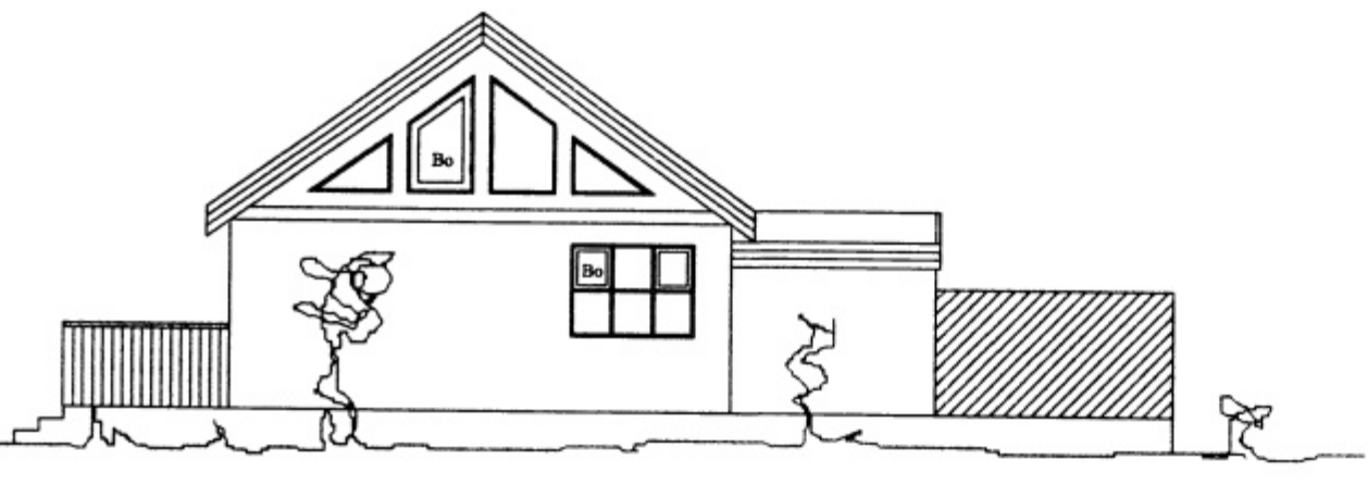
Norðurhlid M 1:100
