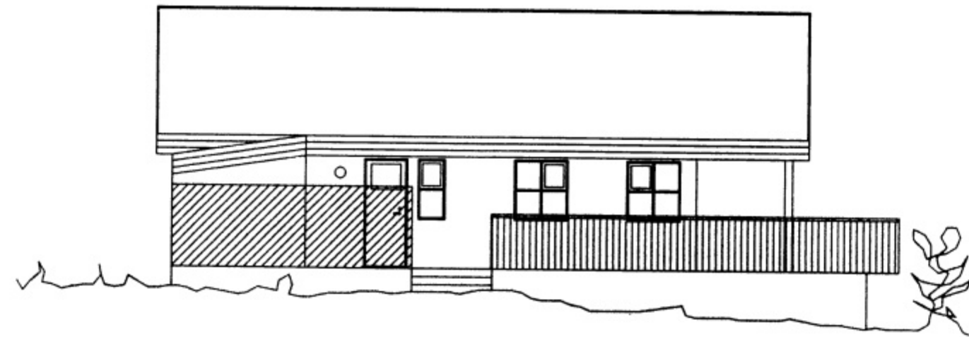
Vesturhlid M 1:100
