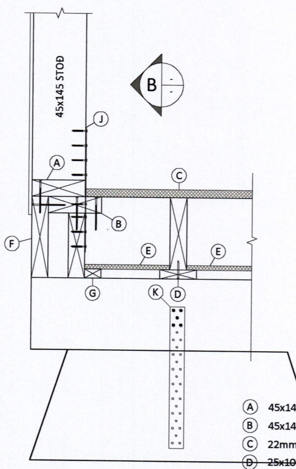
FORSTEYPTAR UNDIRSTÖÐUR
