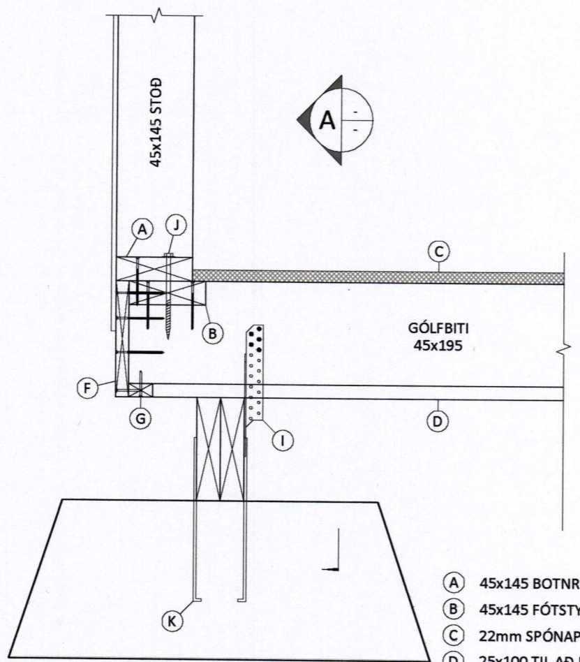
FORSTEYPTAR UNDIRSTÖÐUR
