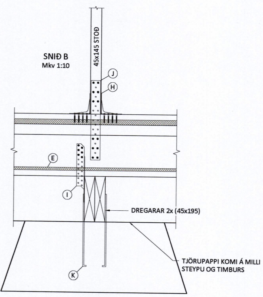
FORSTEYPTAR UNDIRSTÖÐUR
