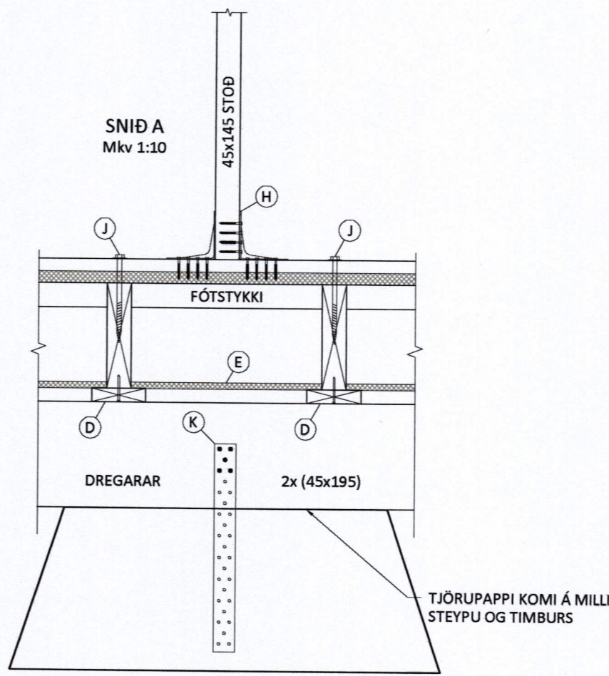
FORSTEYPTAR UNDIRSTÖÐUR
