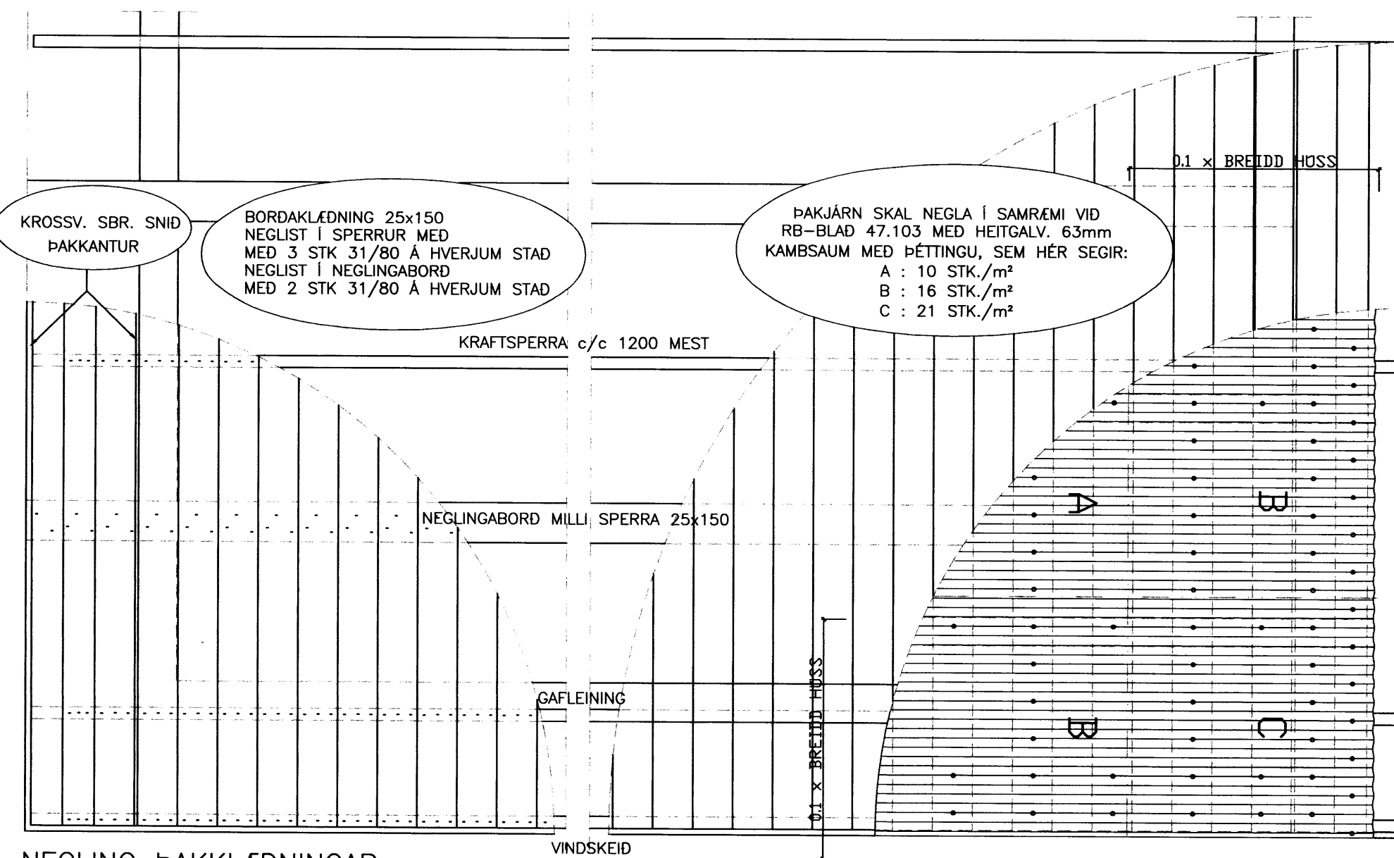
NEGLING ÞAKKLÆDNINGAR MKV. 1:20
