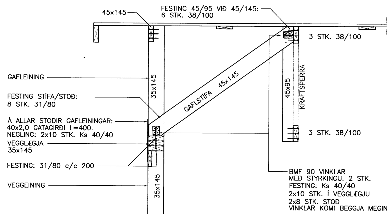
GAFSTIFA MKV. 1:20
