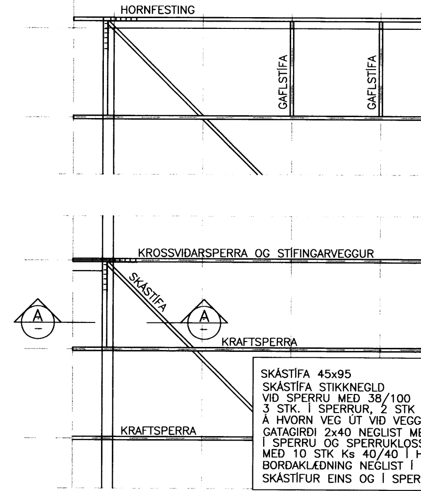
FESTING SKASTIFA Í ÞAKI MKV. 1:50
