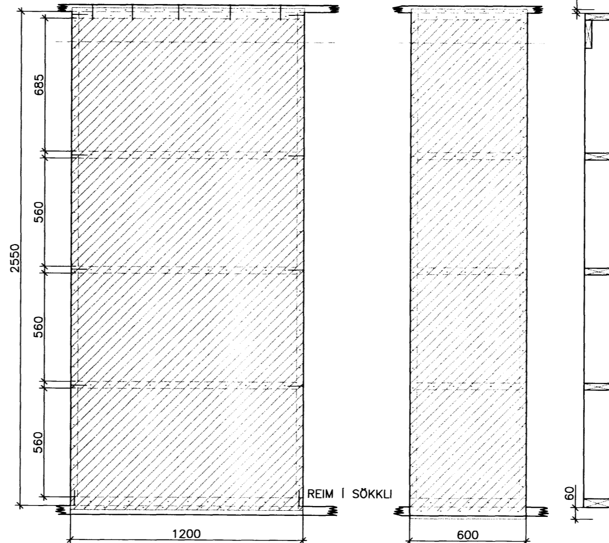
STÍFAR EININGAR MKV. 1:20
