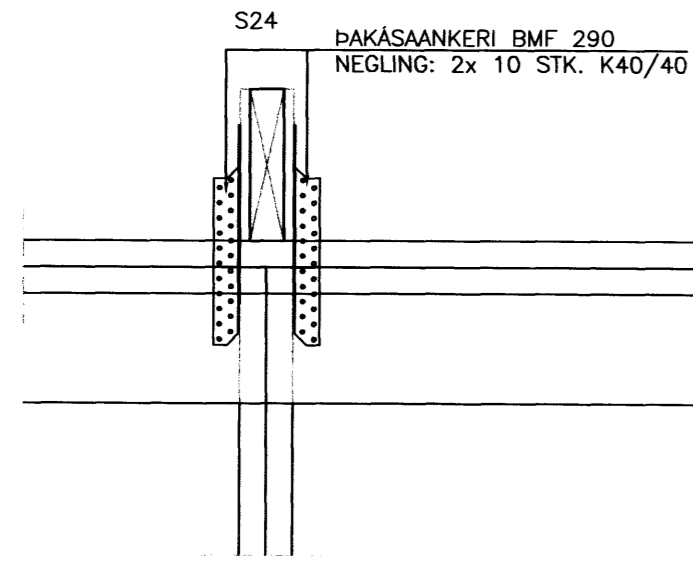
FESTING VIÐ SPERRU S24 Mkv. 1:10
