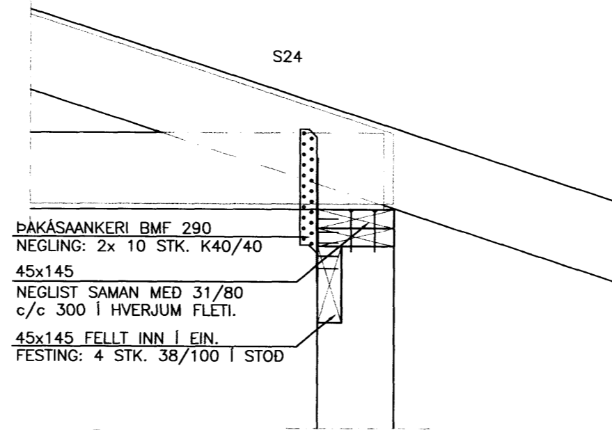
DEILI 1 1:10
