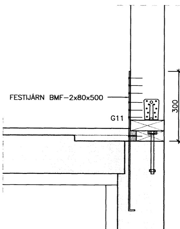
DEILI 1 1:10
