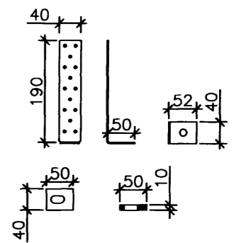
BMF 190x50x2.0x40 VINKILL OG BMF 40x10x50 STEYPUSKINNA MKV. 1:10
