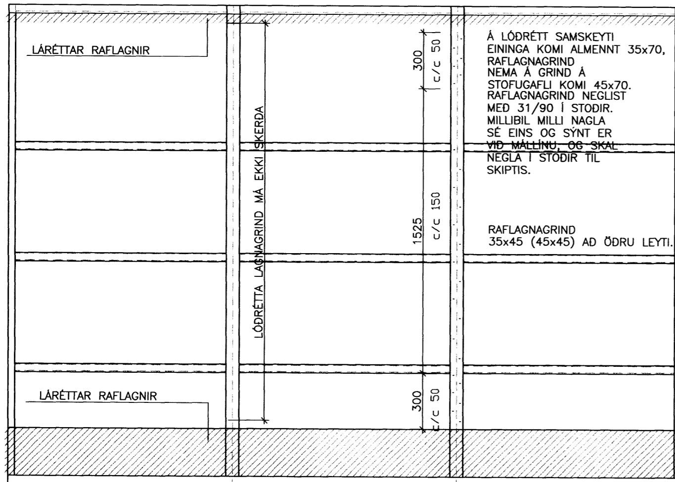
FRÁGANGUR RAFLAGNAGRINDAR Mkv. 1:20
