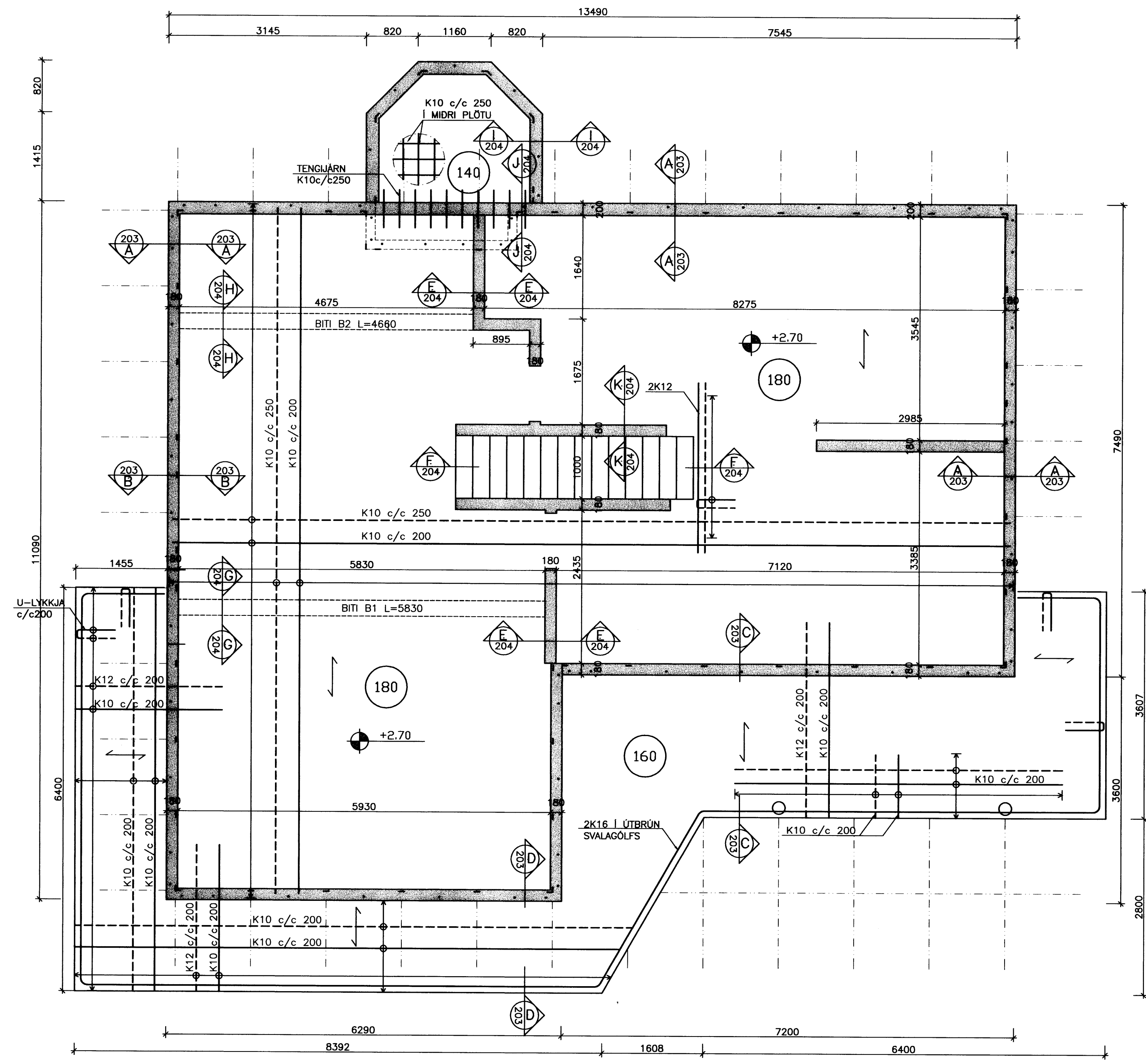
PLATA 2. HÆÐ MKV. 1:50
