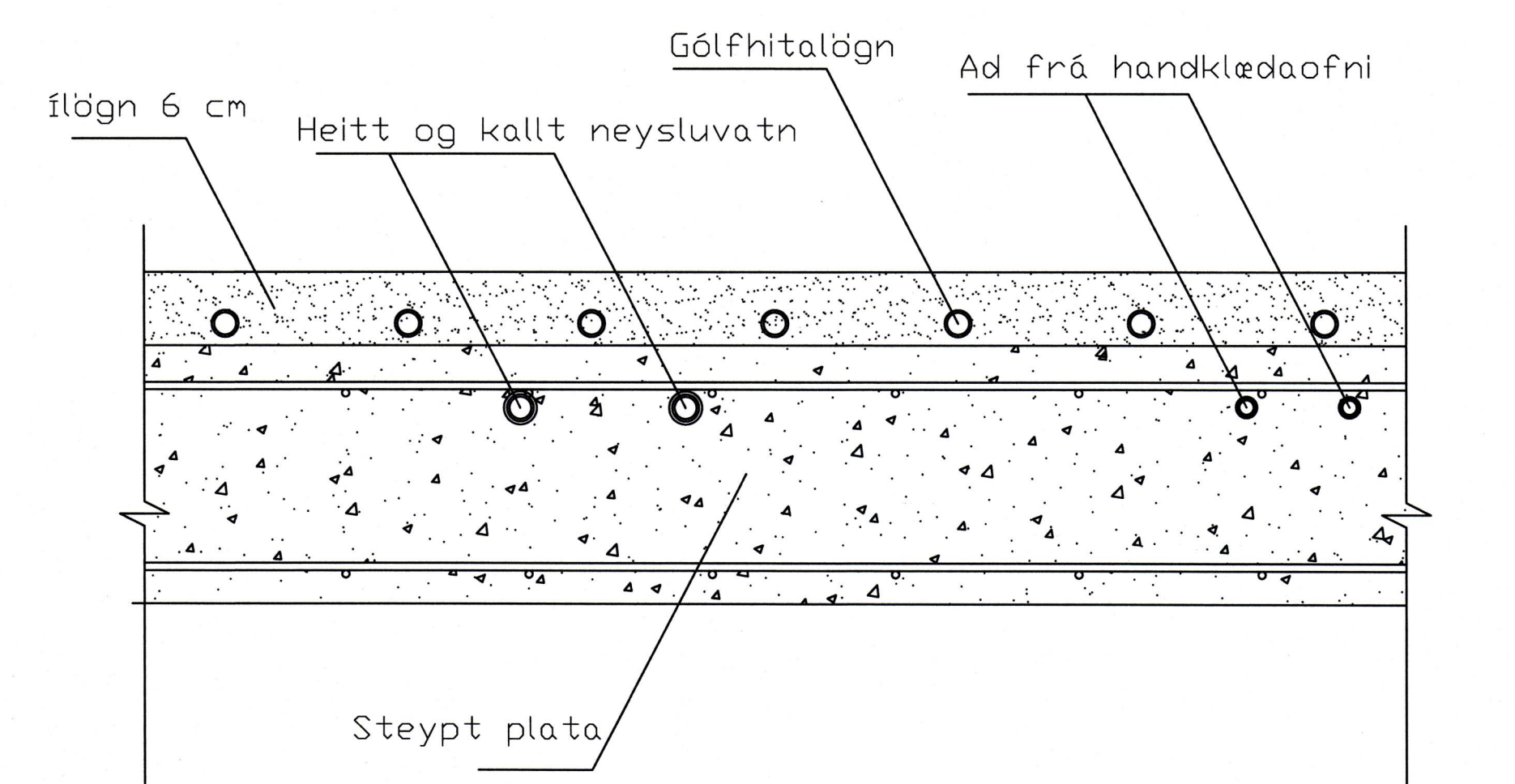
STADSETNING HITA OG VATNSLAGNA Í PLÖTU EFRI HÆÐ
