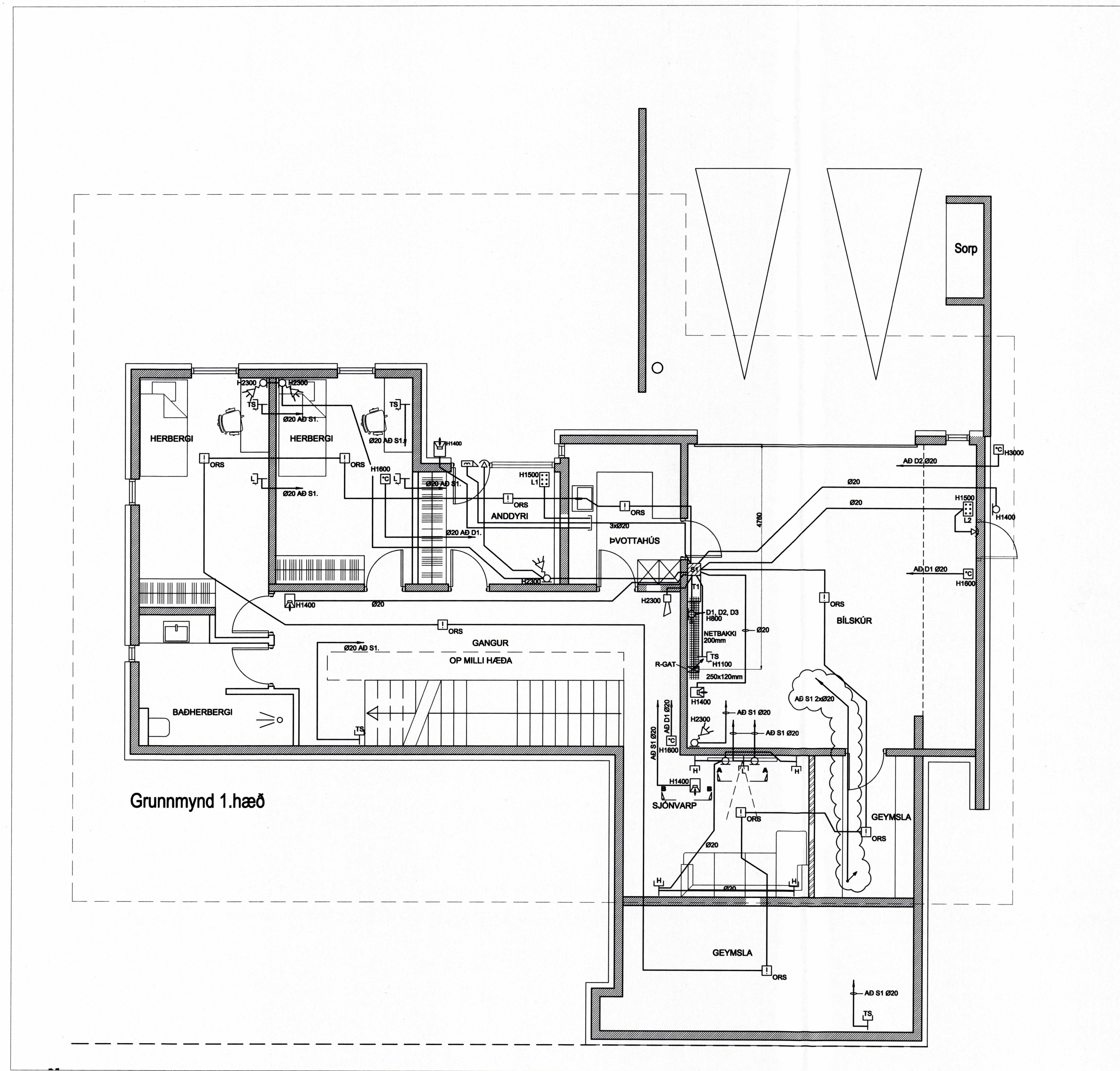
GRUNNMYND 1:50
