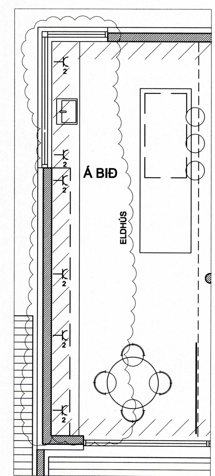
GRUNNMYND ELDHÚS 1:50
