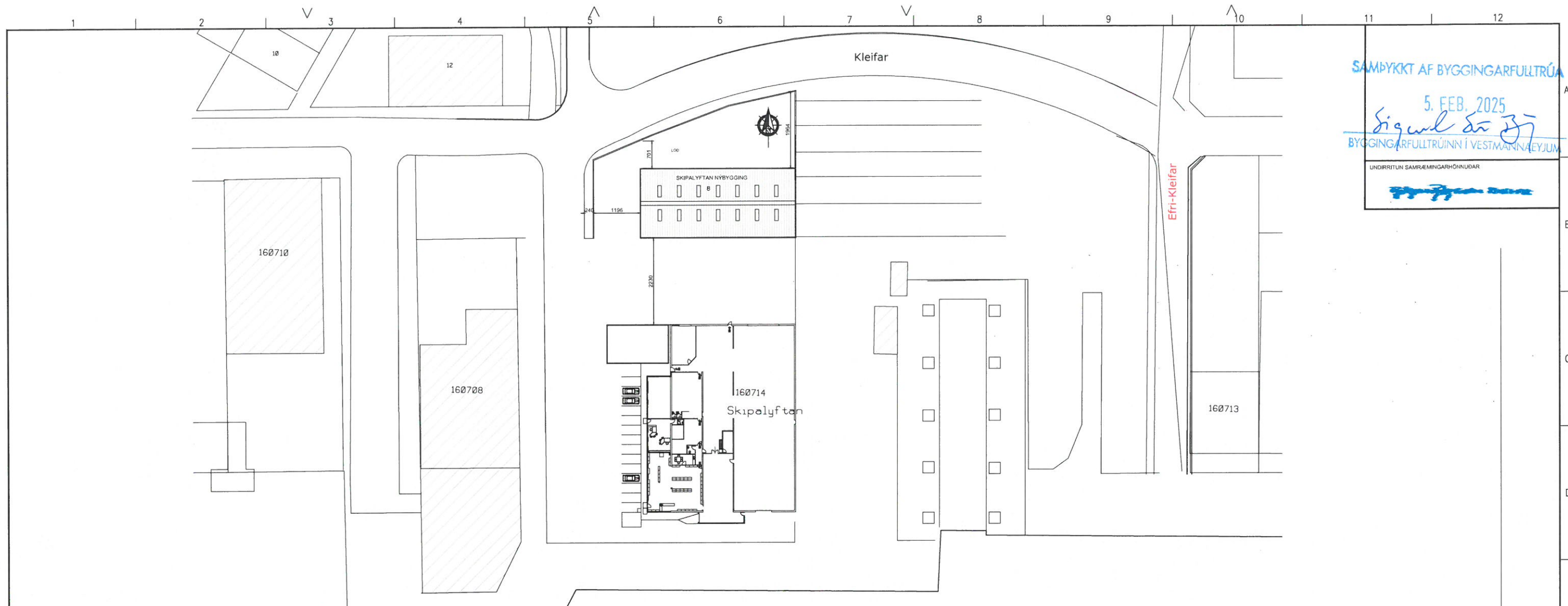
AFSTÖÐUMYND 1:500
