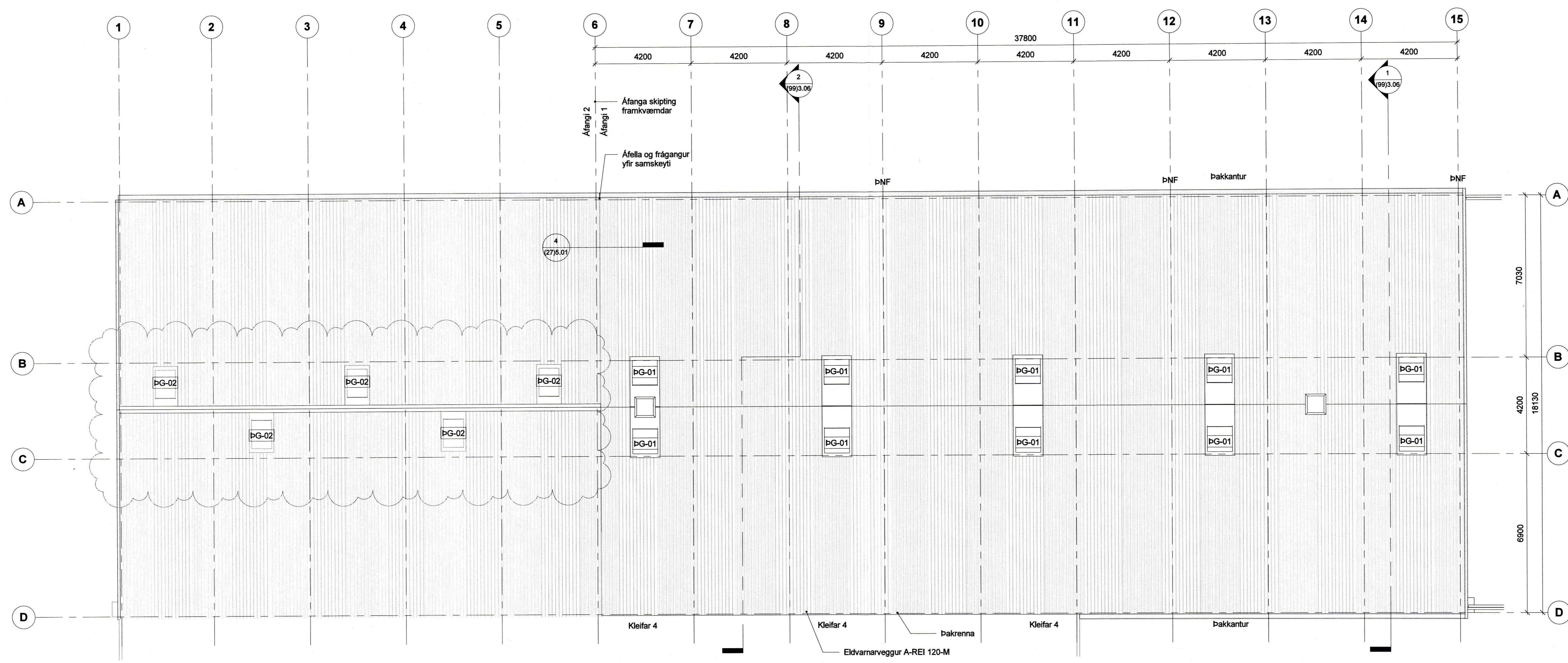
1 (99) Þakmynd 1 : 100
