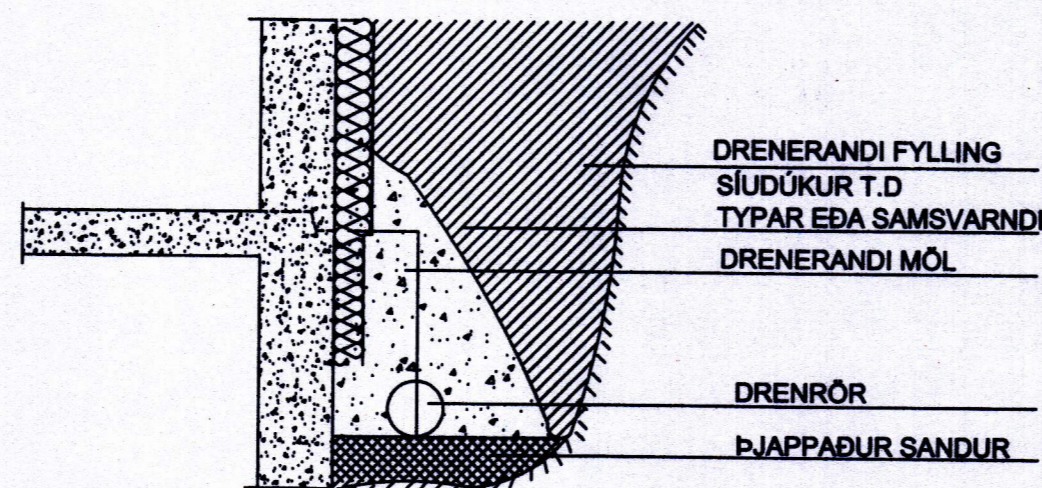
FRÁGANGUR DRENLAGNAR
