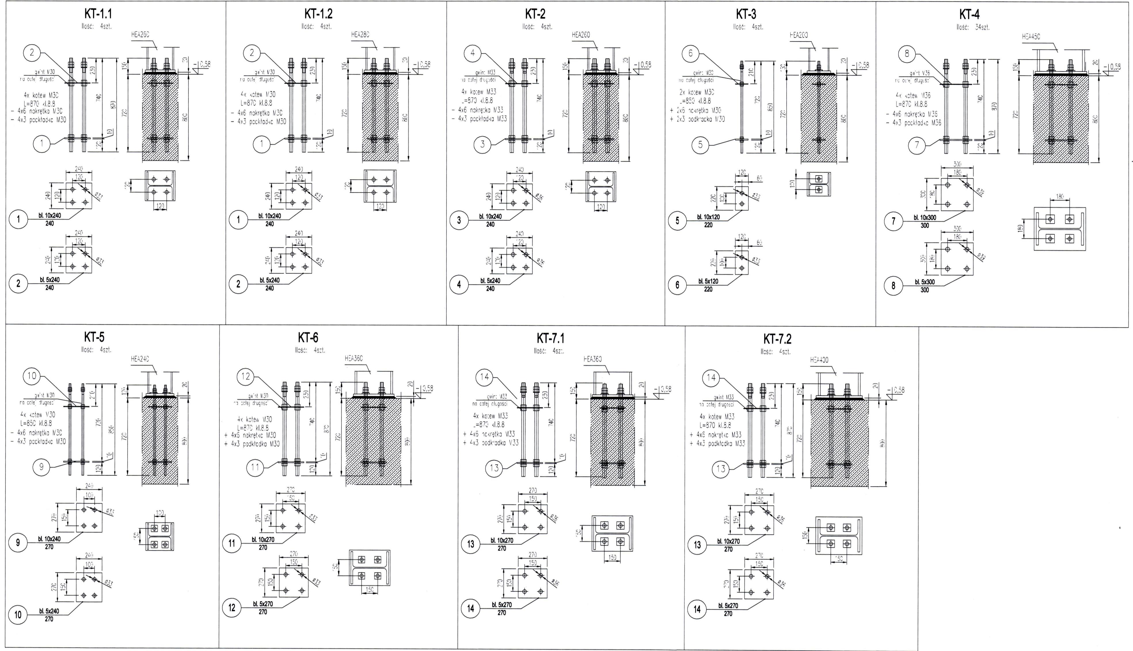
1 Snið Festingar súlur 1 : 20
