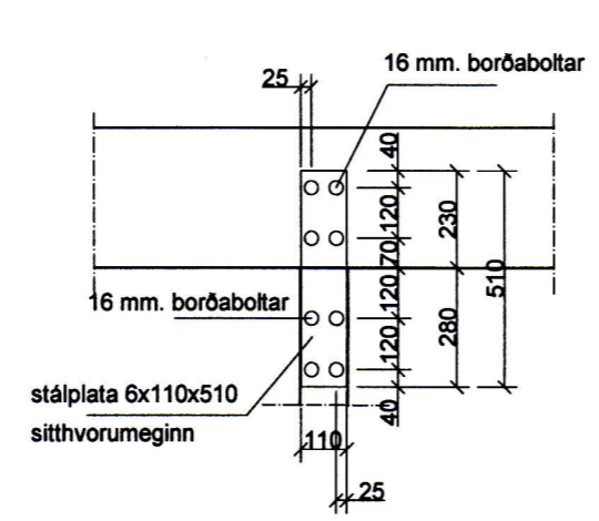
SNIÐ C-C 1:20
