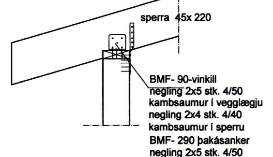
SNIÐ A-A 1:20
