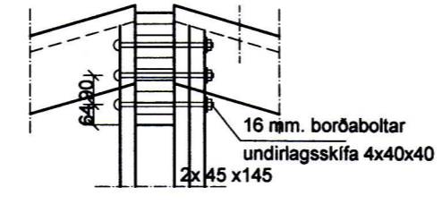
SNIÐ D-D 1:20
