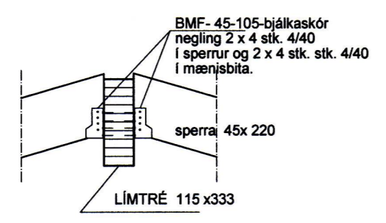
SNIÐ B-B 1:20
