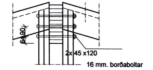
SNIÐ E-E 1:20
