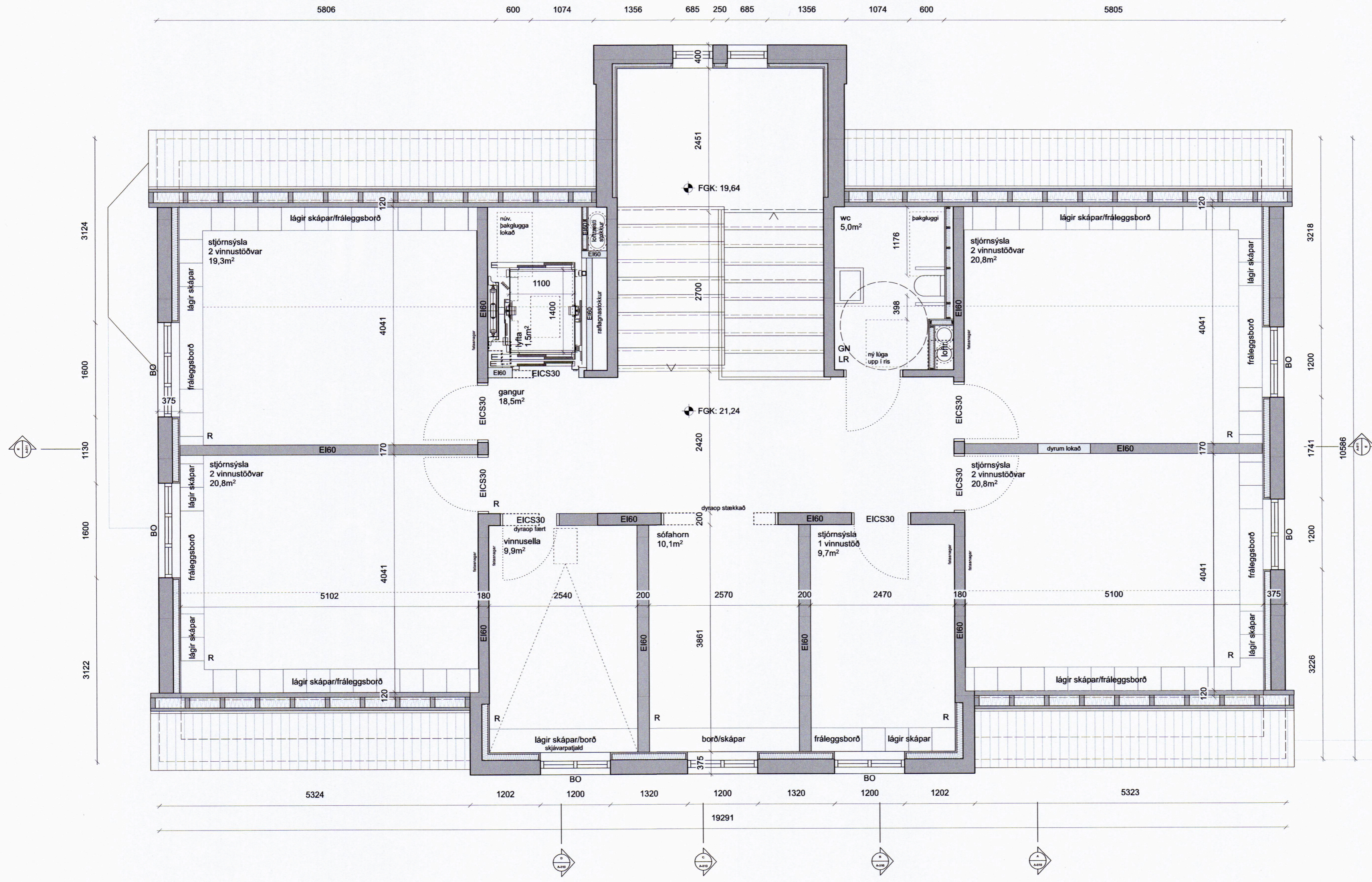
Grunnmynd 2. hæðar
