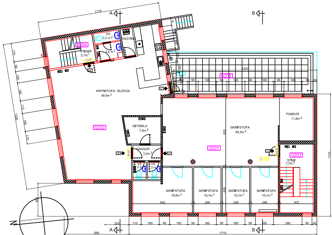
GRUNNMYND 2. HÆÐ 1:100
