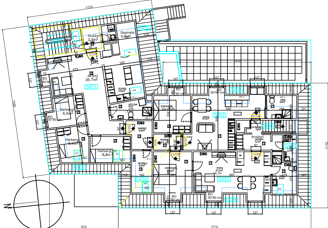
GRUNNMYND 4. HÆÐ 1:100
