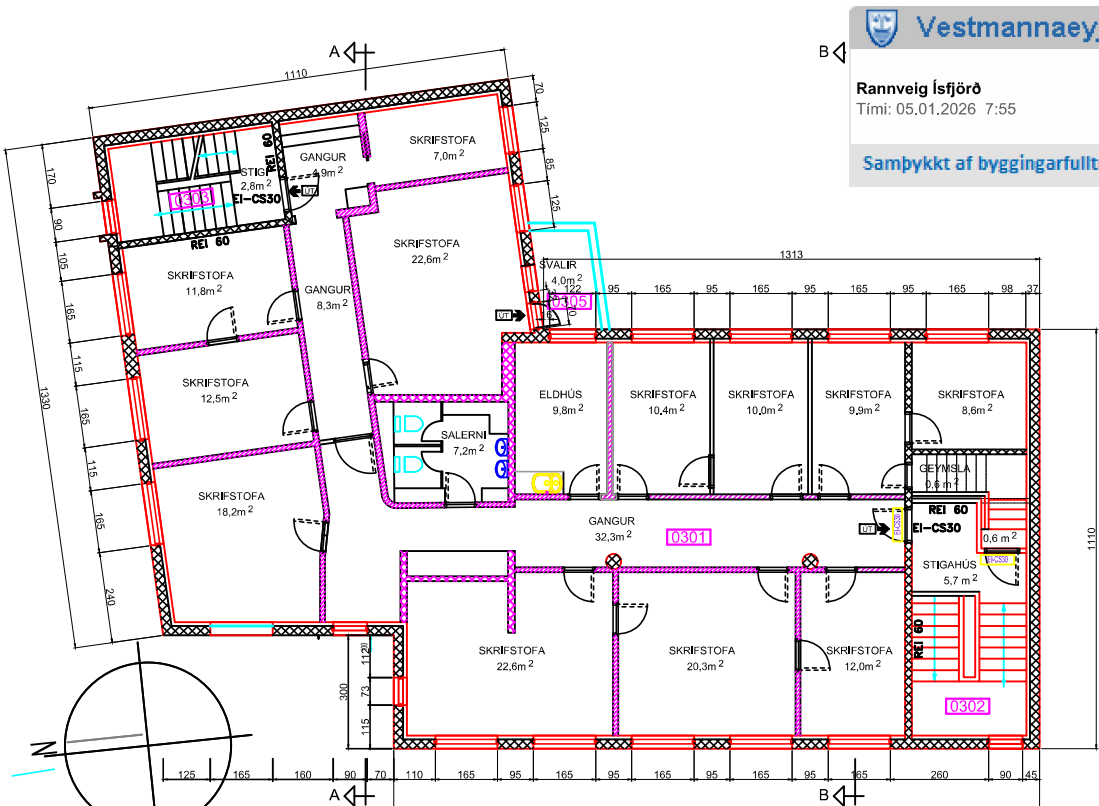
GRUNNMYND 3. HÆÐ 1:100
