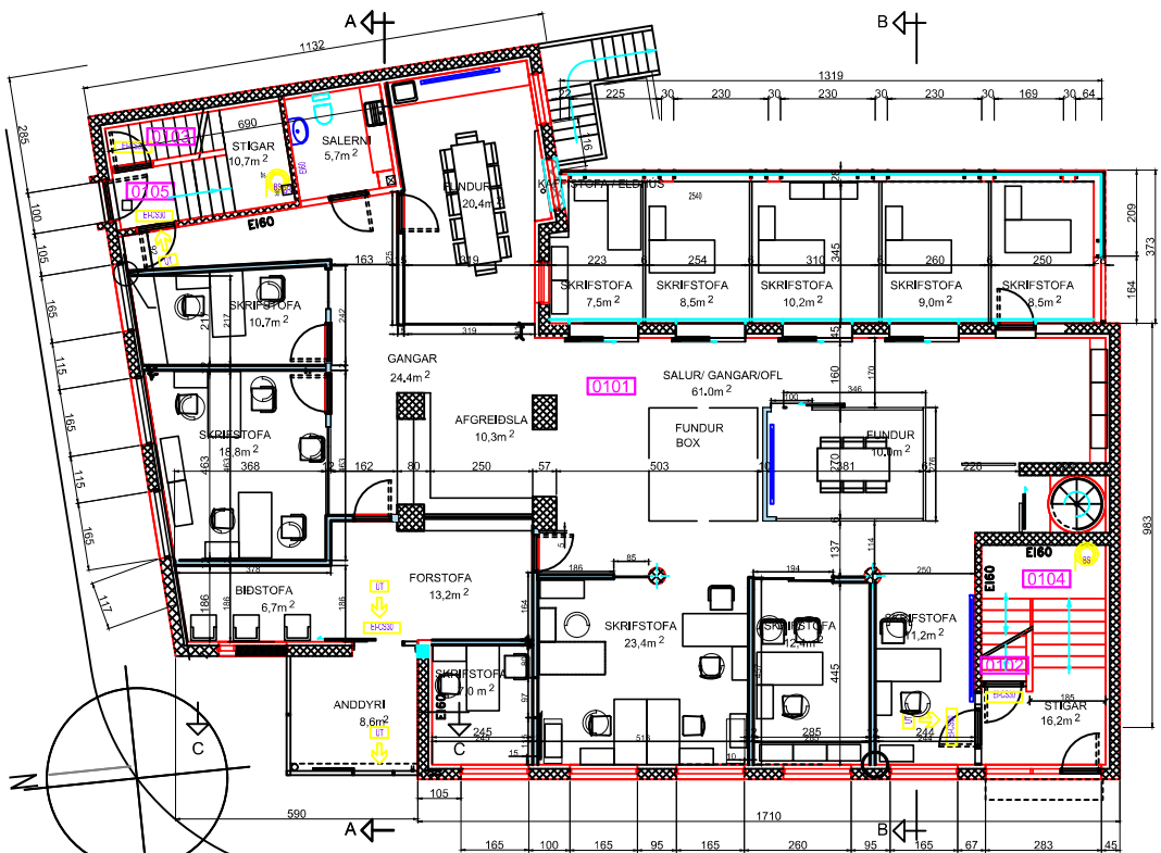
GRUNNMYND 1. HÆÐ 1:100
