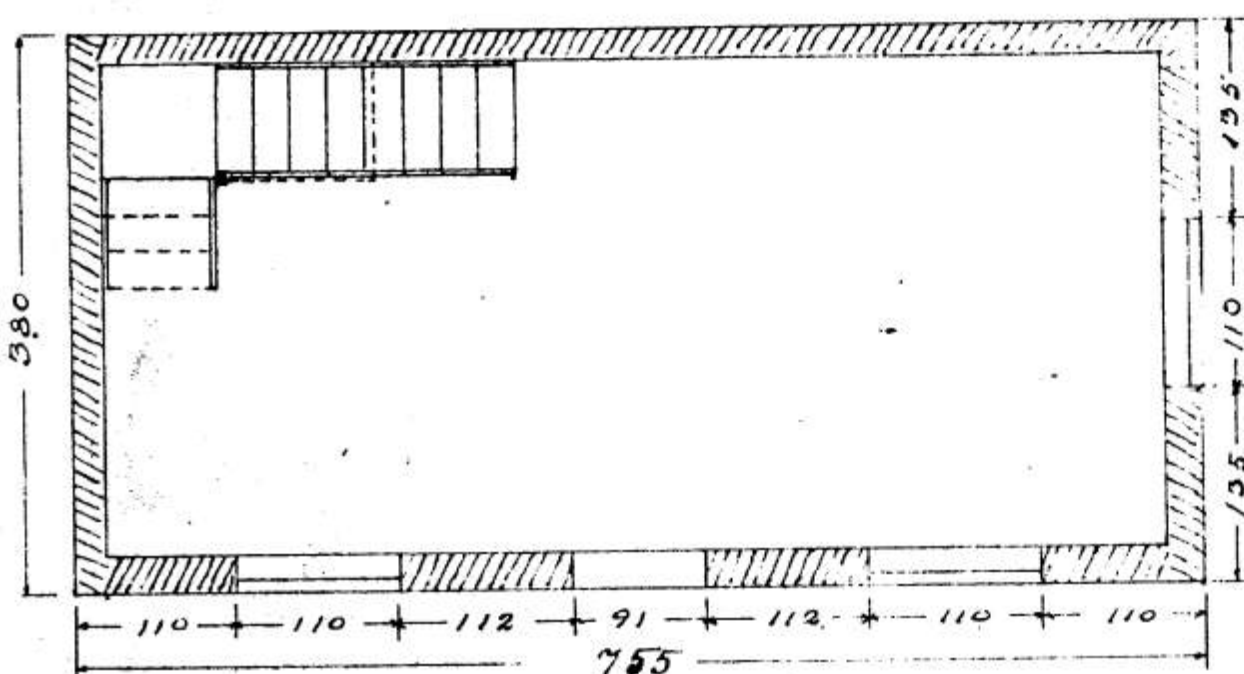
Grunnflötur
