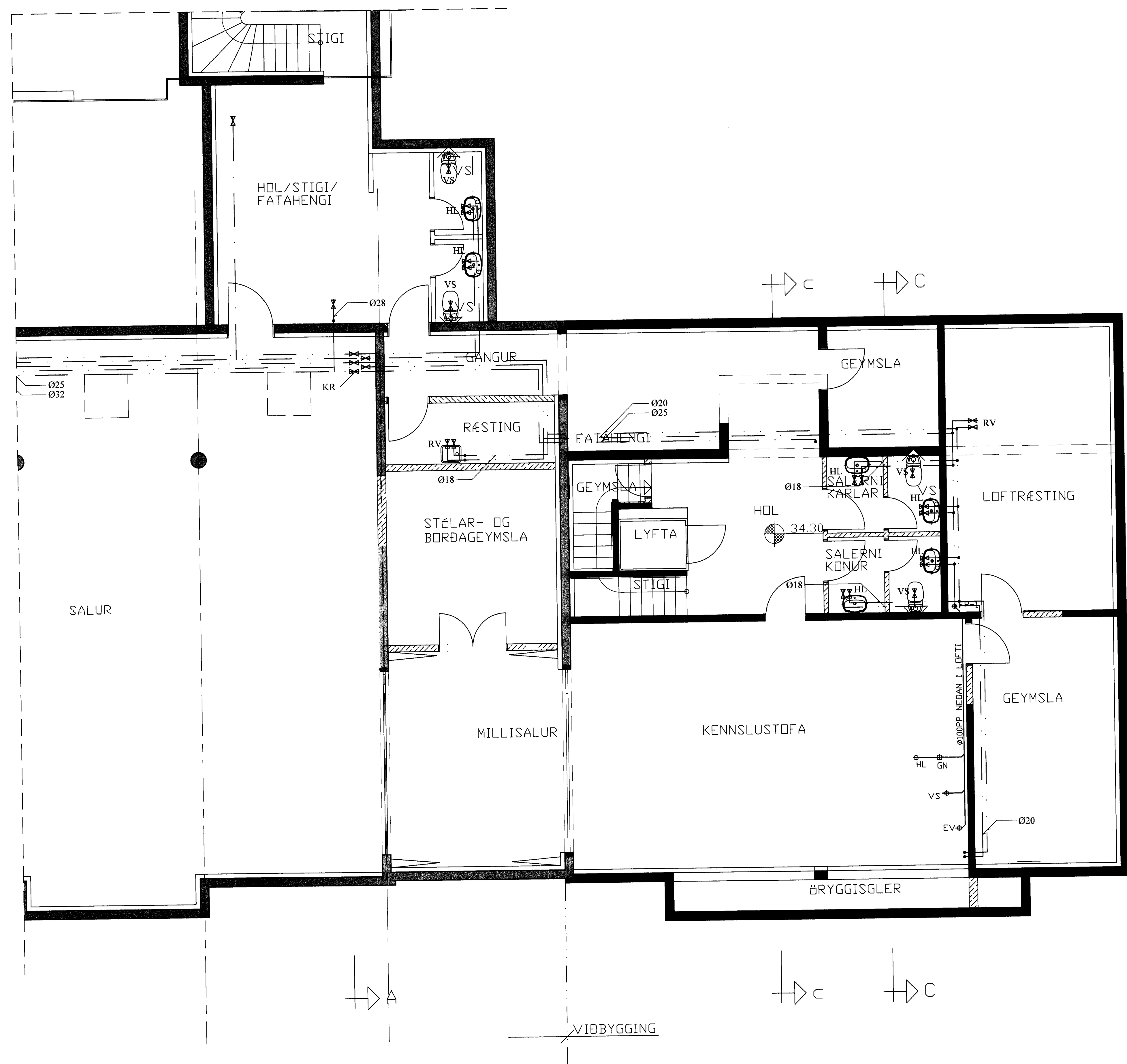
GRUNNMYND VESTURENDI M=1:50
