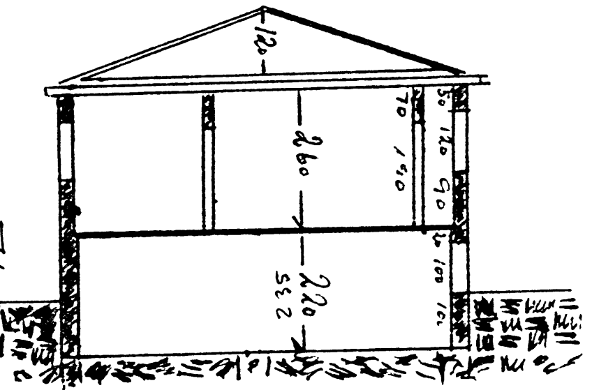
SKURÐUR A-B.
