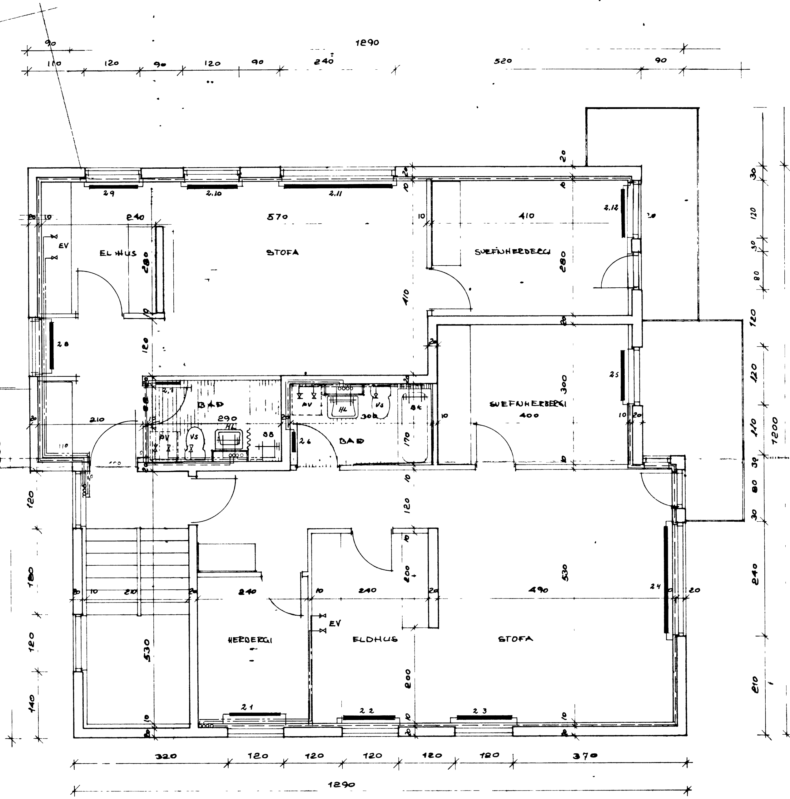
GRUNNMÝND 2 HÆÐ 150
