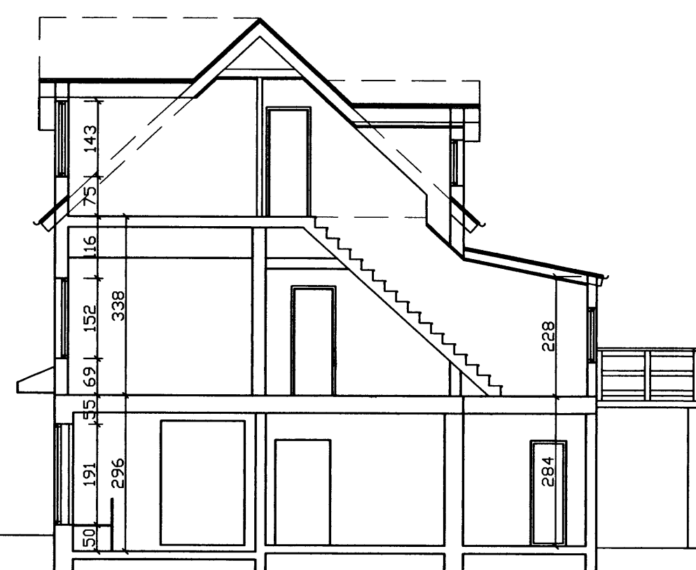
SNIÐ A-A
