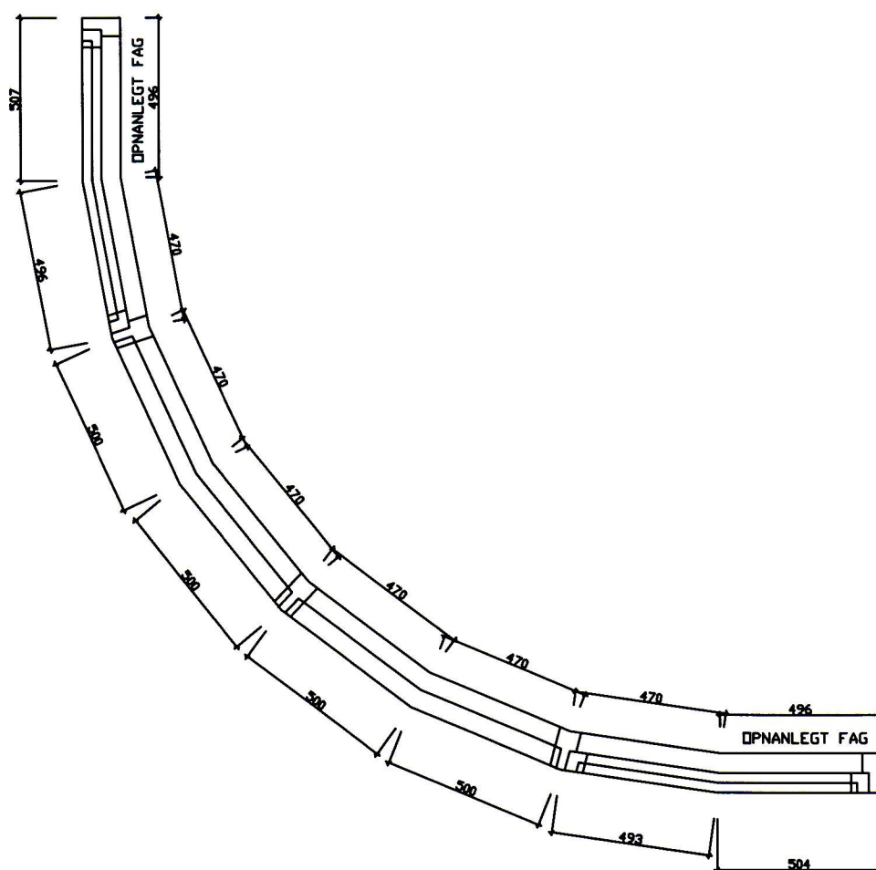
GLUGGI 1 STK.
