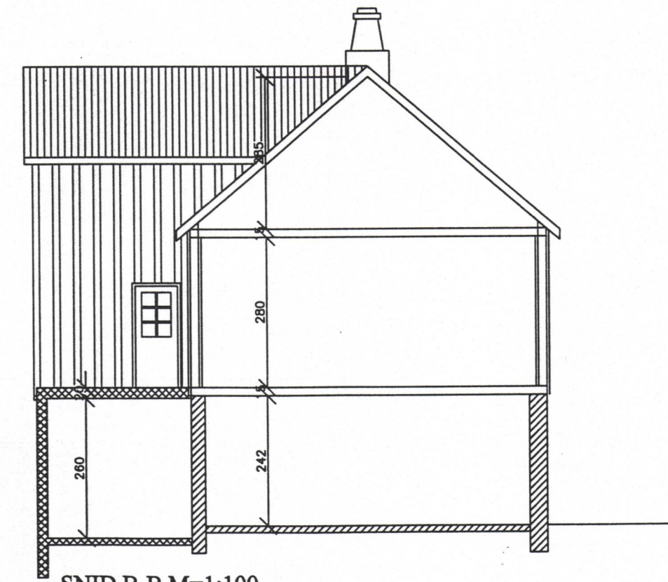
SNID B-B M=1:100
