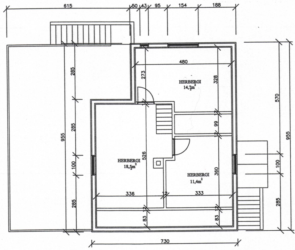
GRUNNMYND RIS M=1:100
