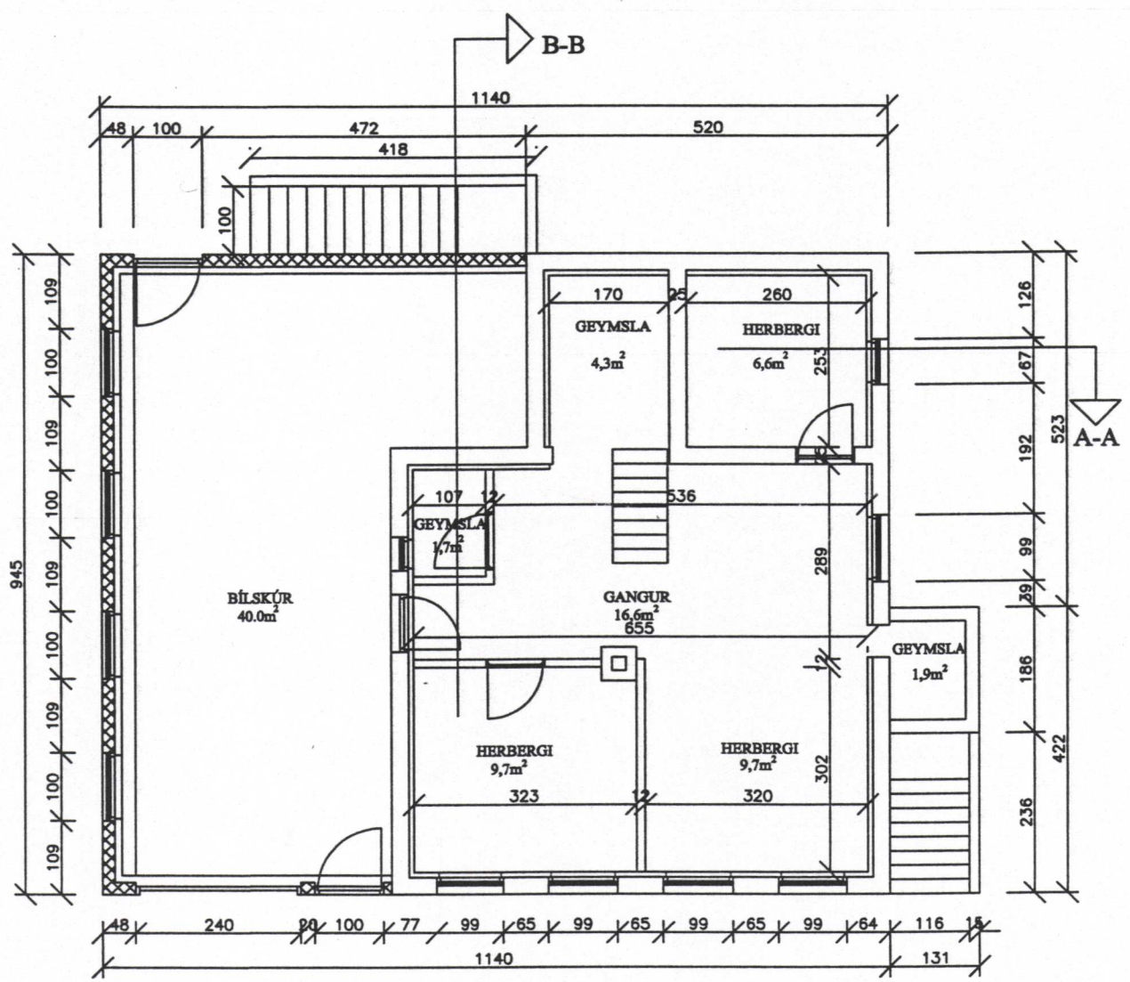
GRUNNMYND KJALLARI M=1:100
