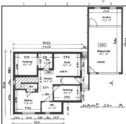
Grunnmynd kjallara 1:100
