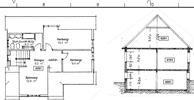
Grunnmynd 2. hæð 1:100
