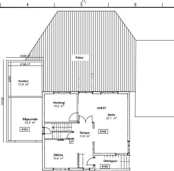
Grunnmynd 1. hæð 1:100
