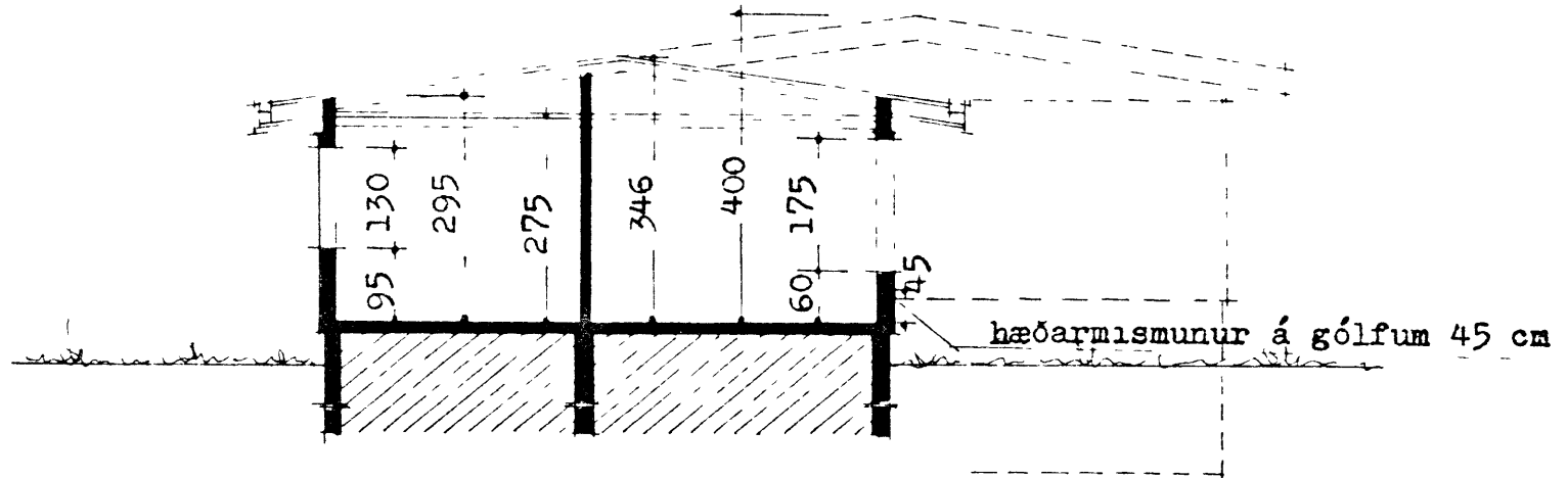
Skurður A-A
