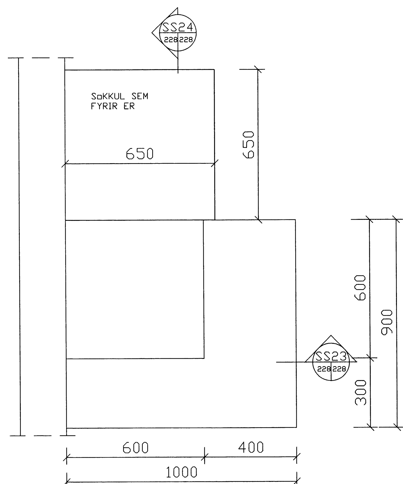
GRUNNMYND VIÐ TENGI BYGGINGU SÄKKUL NR. 3
