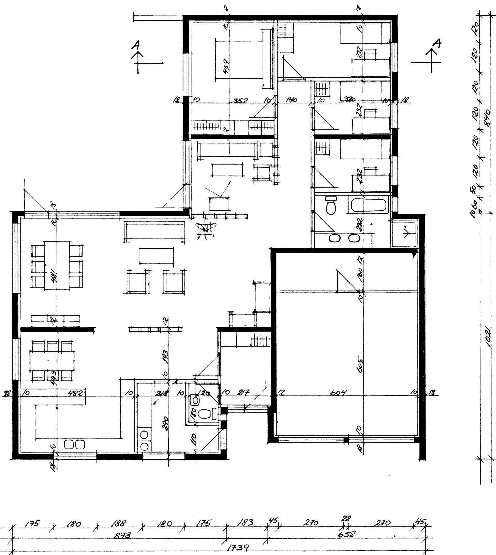
GRUNNMYND 1:100
