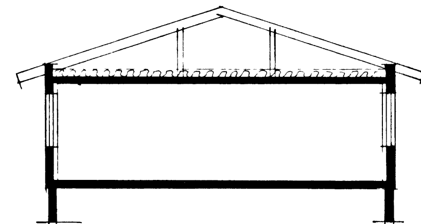
SNID A-A 1:100
