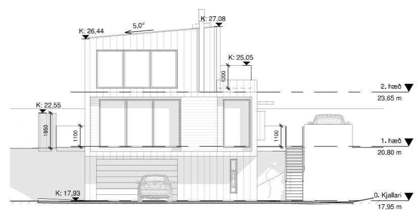
4 Norður 1 : 100
