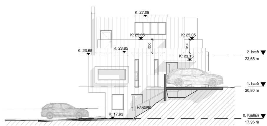
6 Vestur 1 : 100
