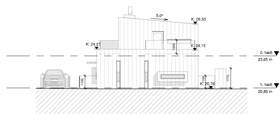
5 Suður 1 : 100
