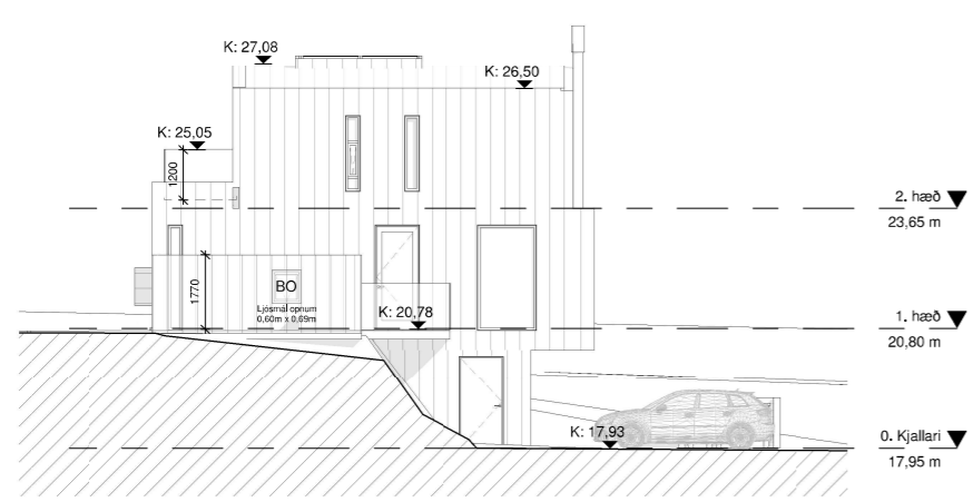
3 Austur 1 : 100
