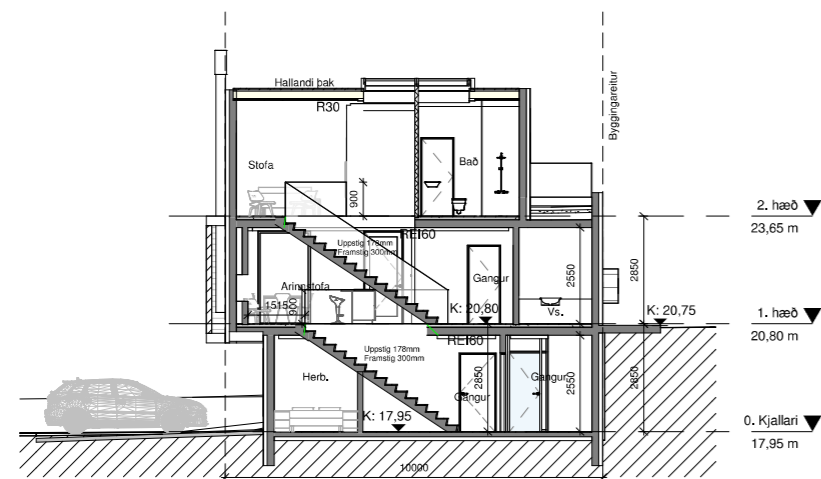
1 Langsnið 1 : 100
