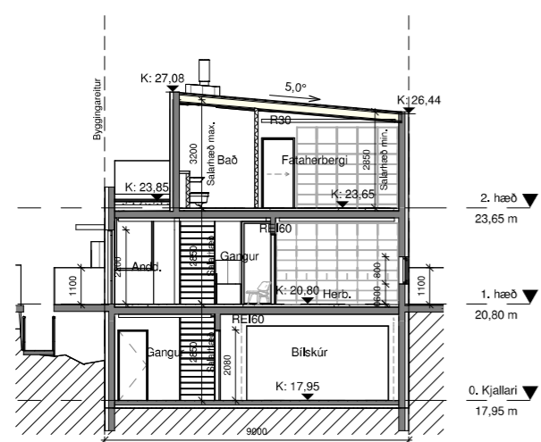
2 Þversnið 1 : 100
