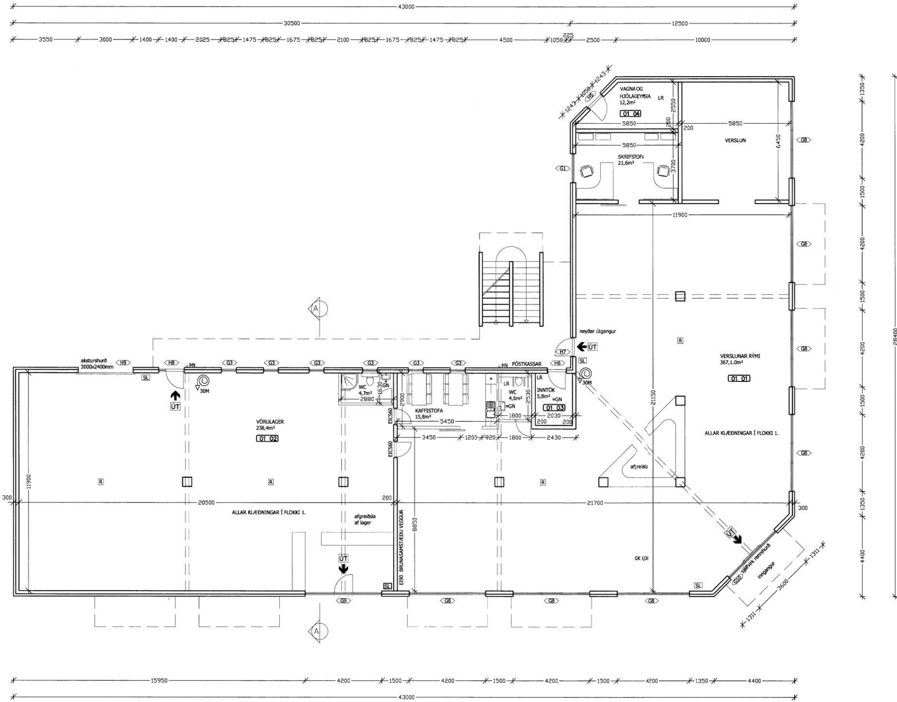
GRUNNMYND 2.HÆÐ 1:100
