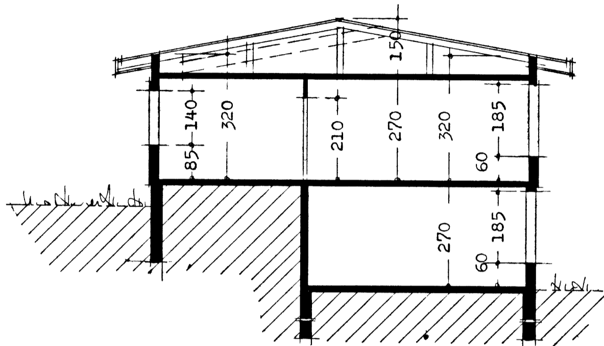
skurður A-A
