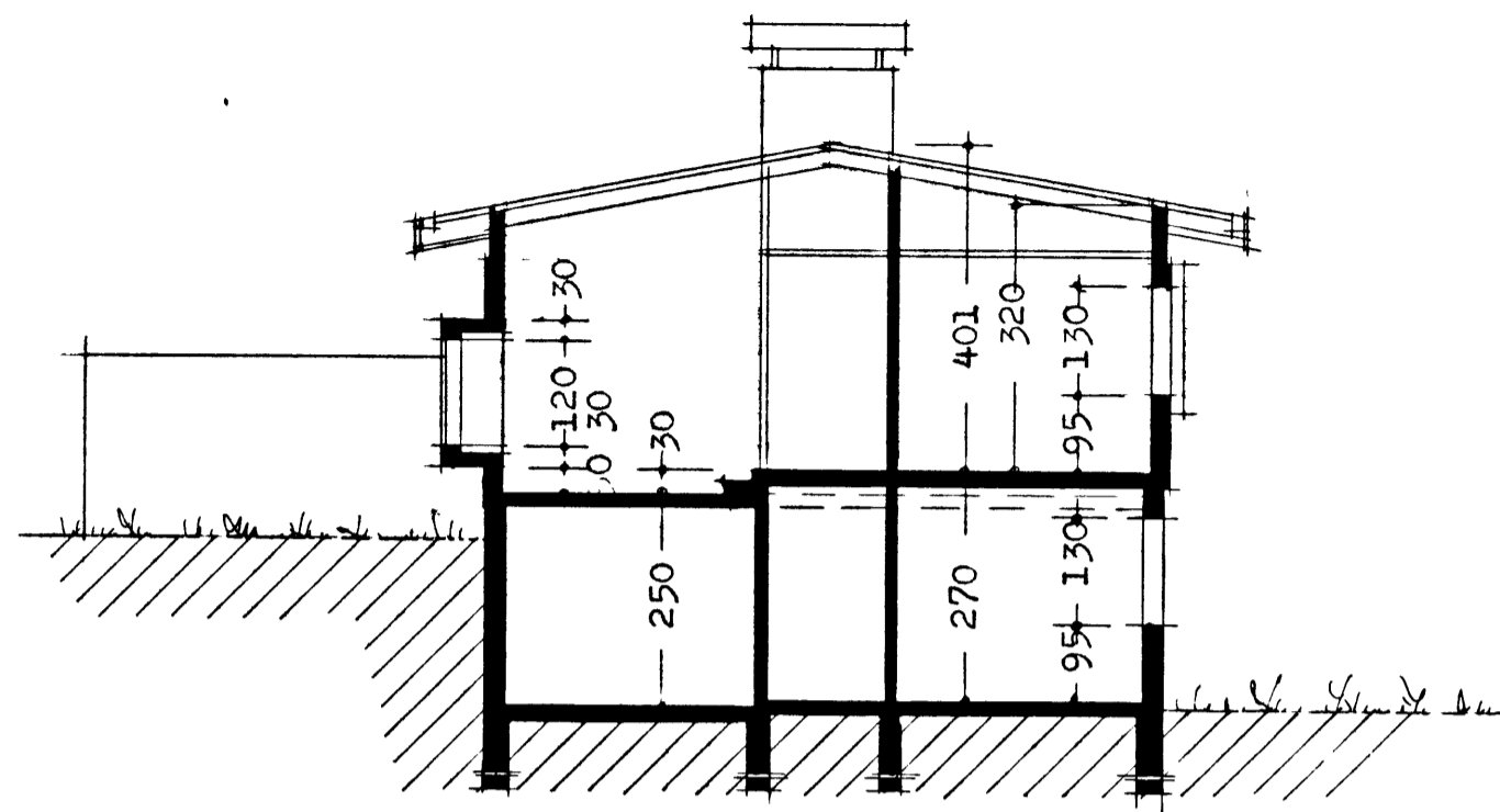
skurður B-B
