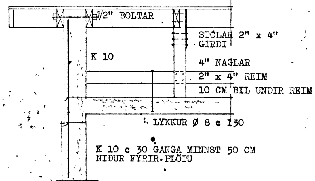
SNID - B 1:20 Í GAFLVEGG
