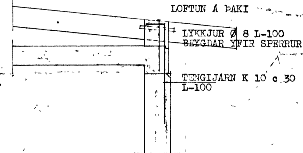
SNID - C 1:20
