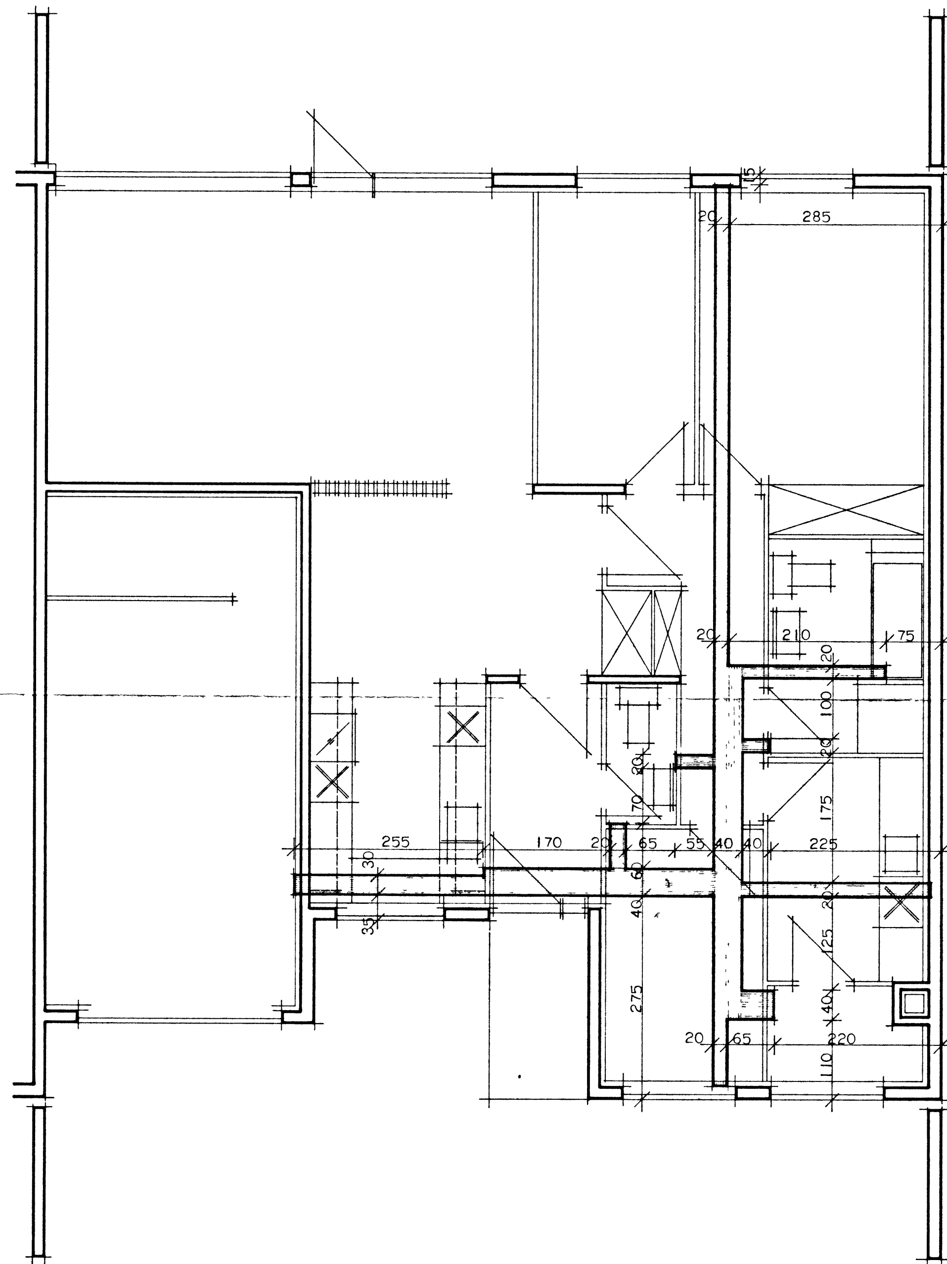
GRUNNMYND GÓLFRAUFA.
