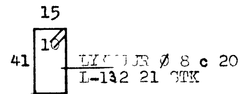
SNID - D 1:20 I HLIÐANV. VÍÐ FLÖTU
