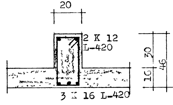
SNID - E 1:20
