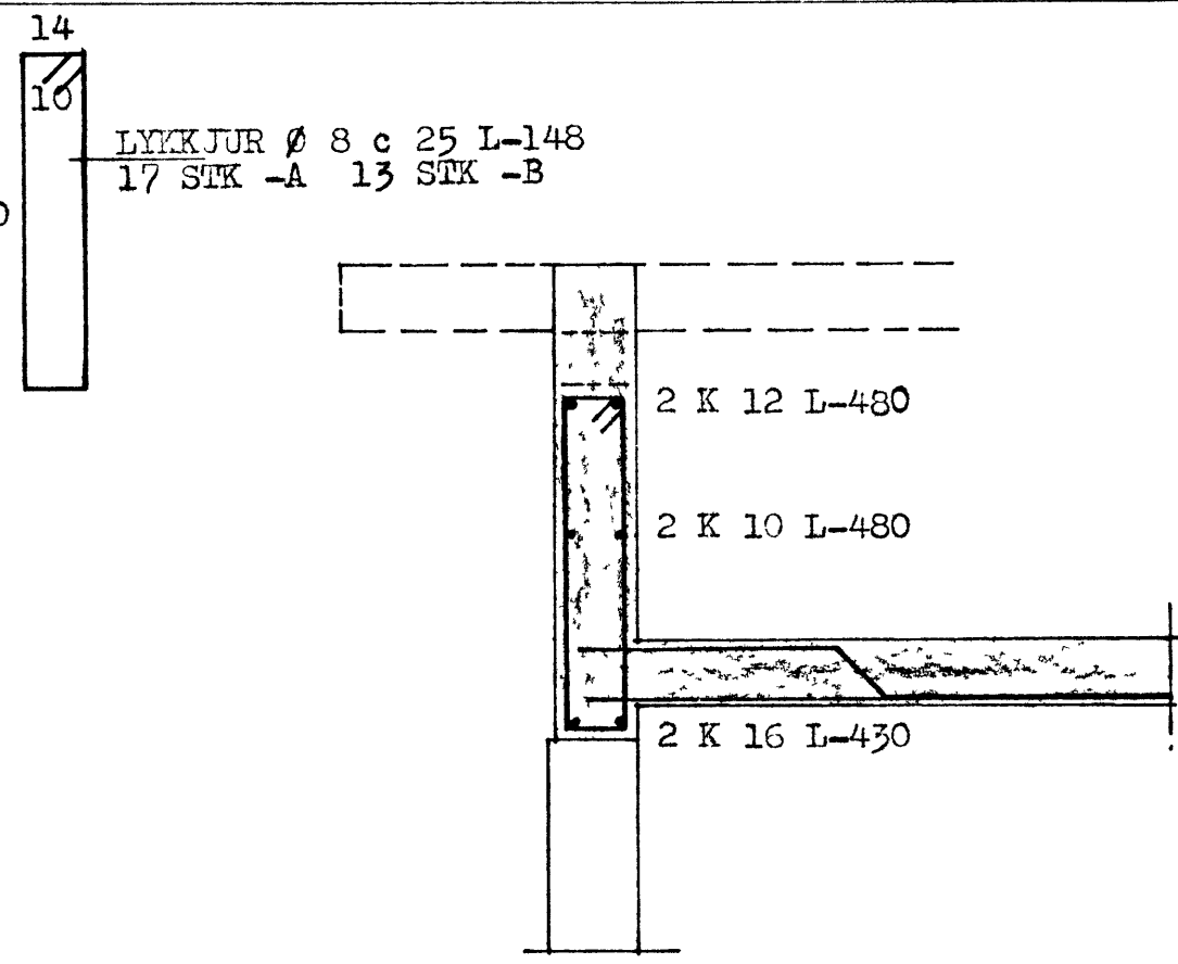
SNID - B 1:20
