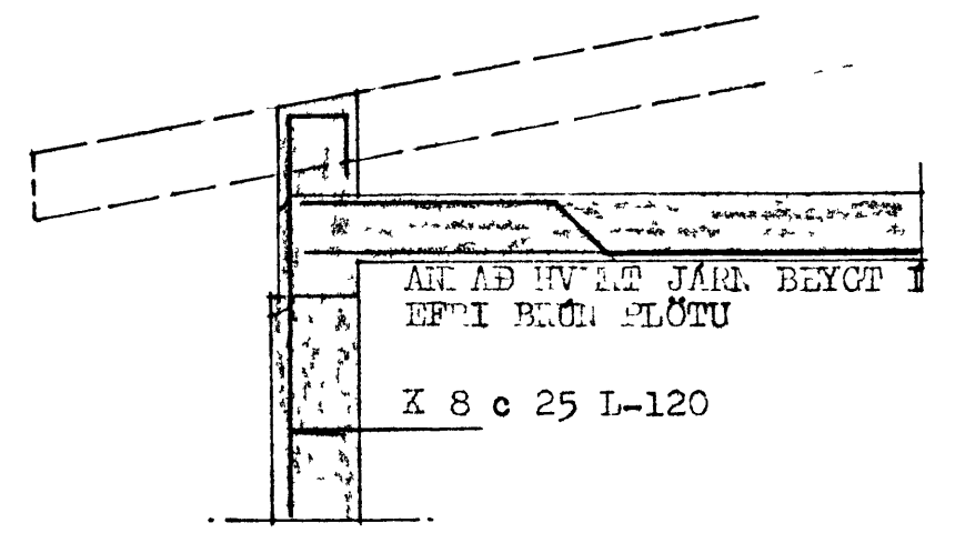
SNID - D 1:20 I HLIÐANV. VÍÐ FLÖTU
