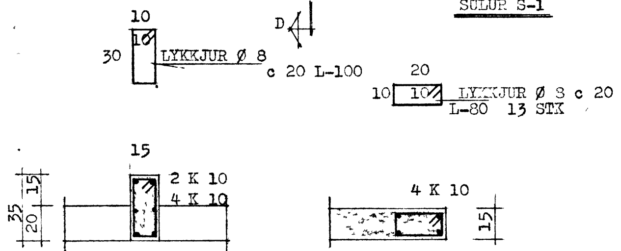
SÚLA S-1 1:20
