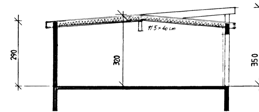
SNIÐ
