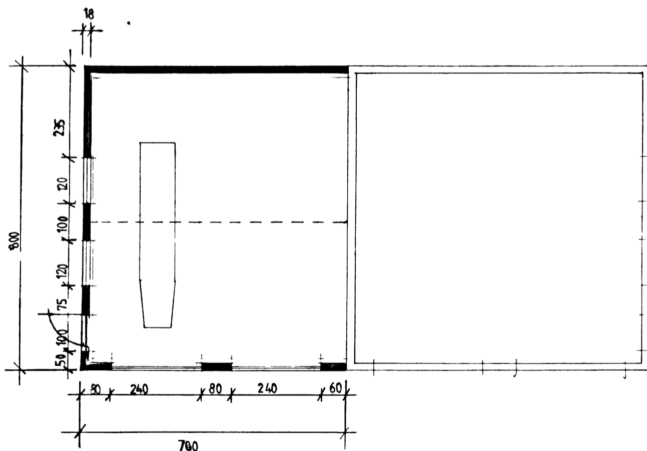
GRUNNMYND
