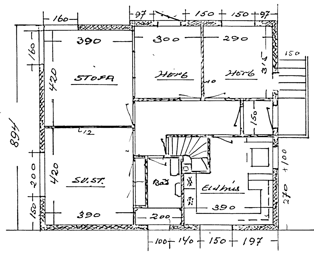
1 HÆÐ
