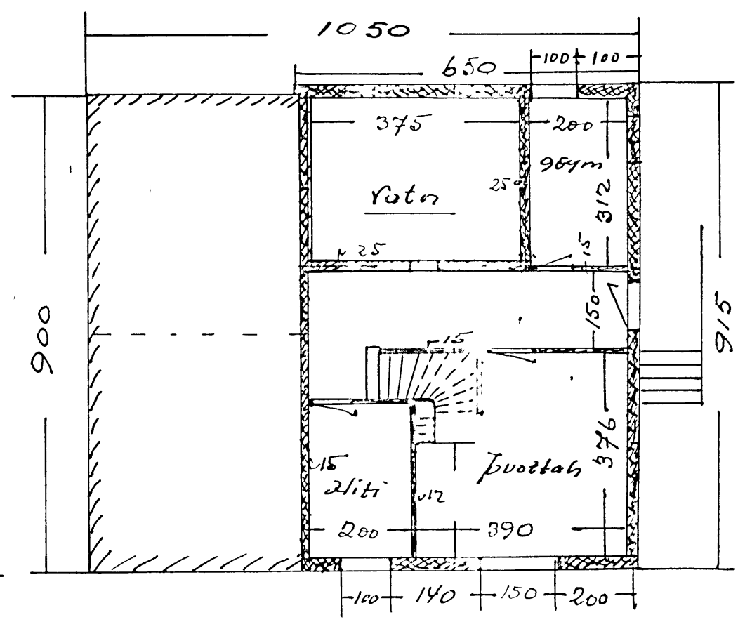
2 HÆÐ
