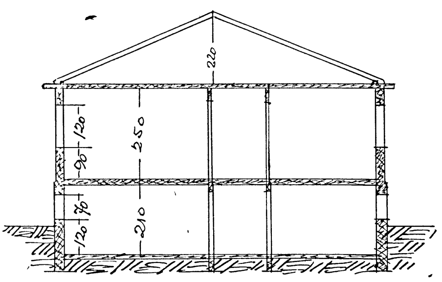
SKURÐUR
