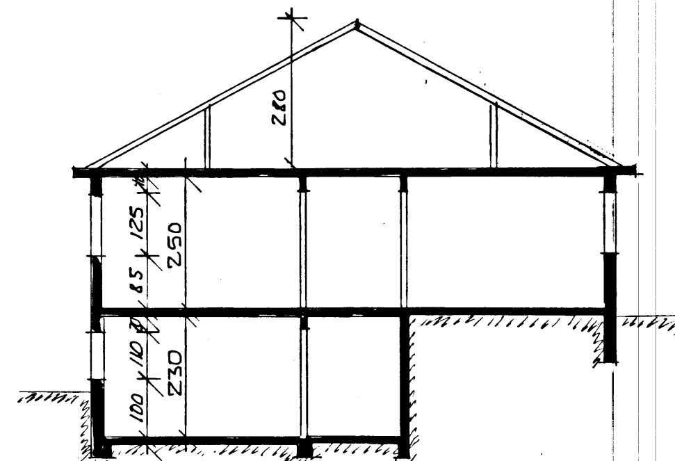
SKURÐUR M=1:100
