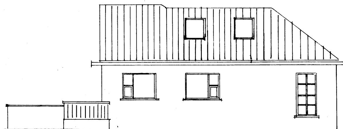
SUÐURHLIÐ M=1:100
