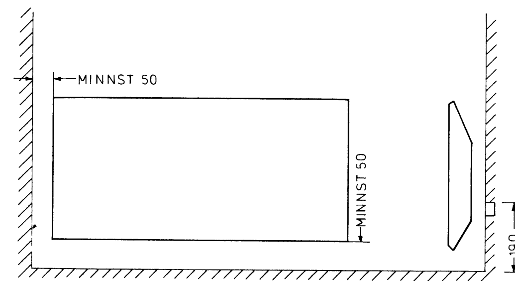
Frágangur ofna á vegg (mál í mm)
