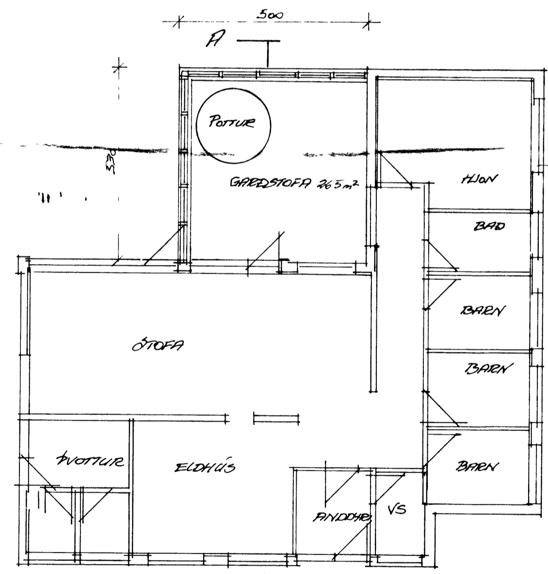
GRUNNMUND
