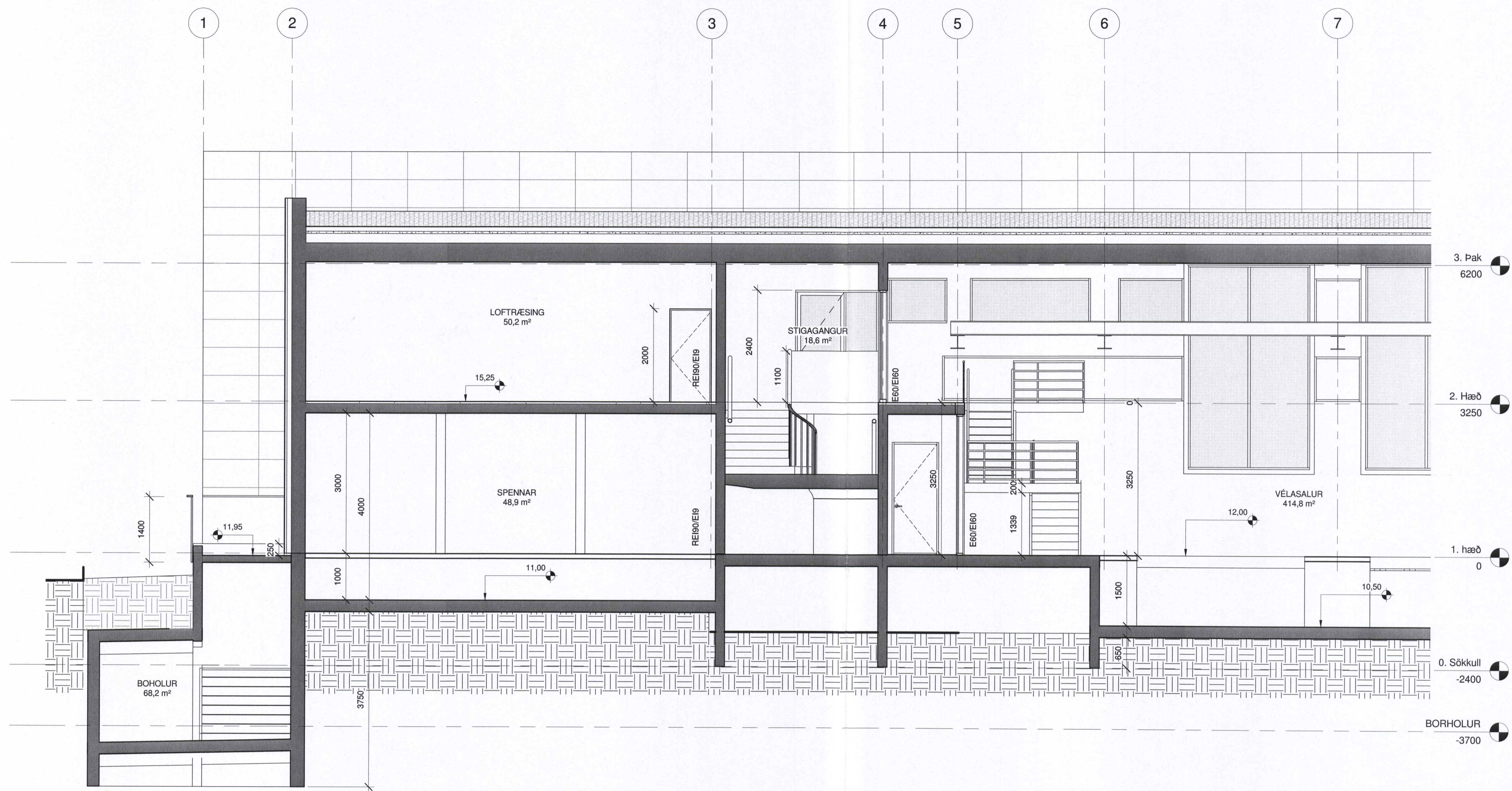
D-E LANGSNIÐ NORÐURENÐI 1 : 50
