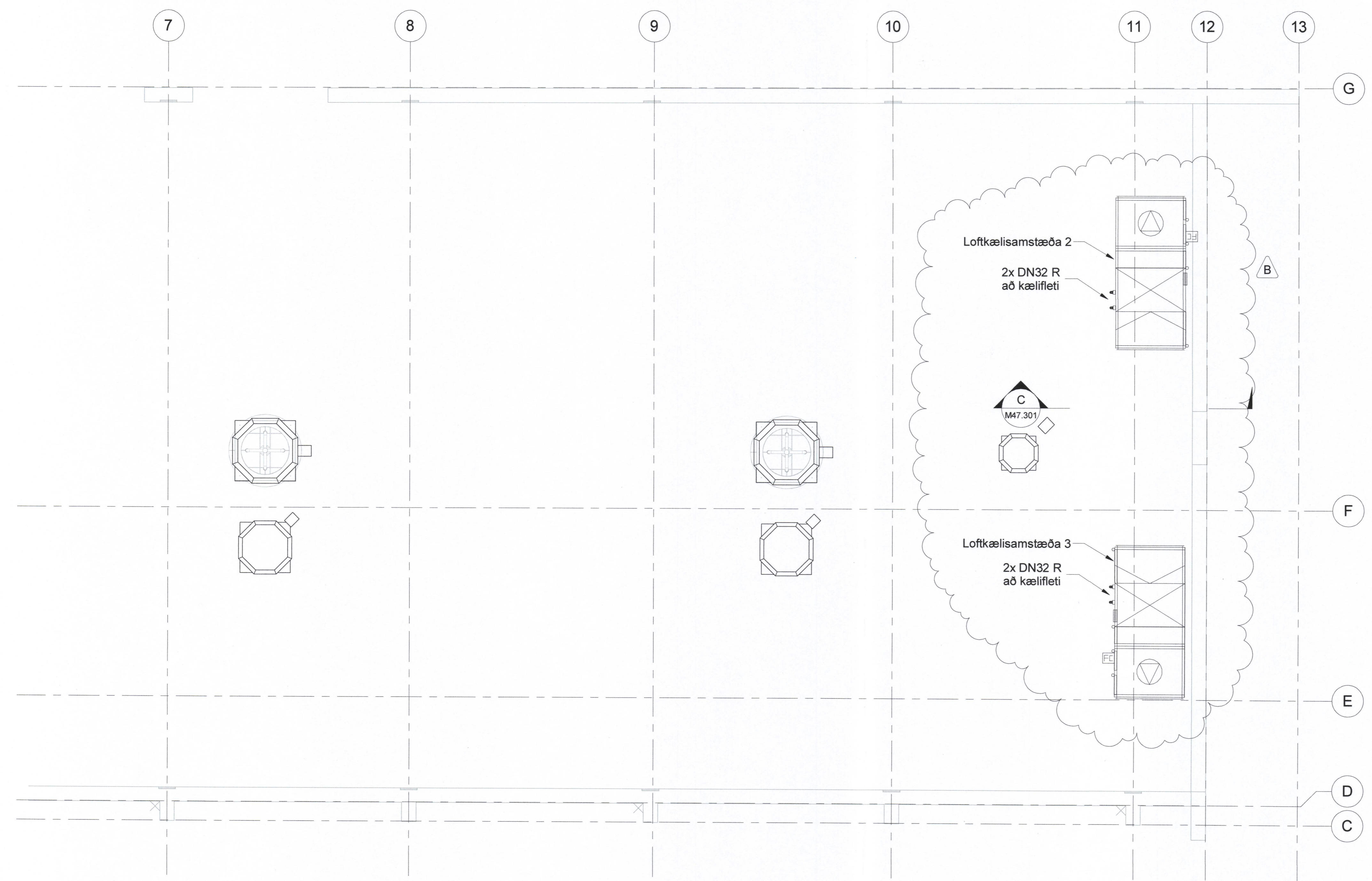
GRUNNMYND 2. HÆÐ 2/2 1 : 50
