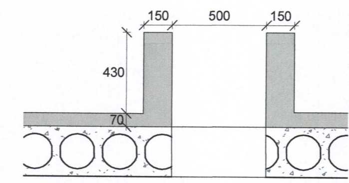
2 SNID C50.107 1 : 20
