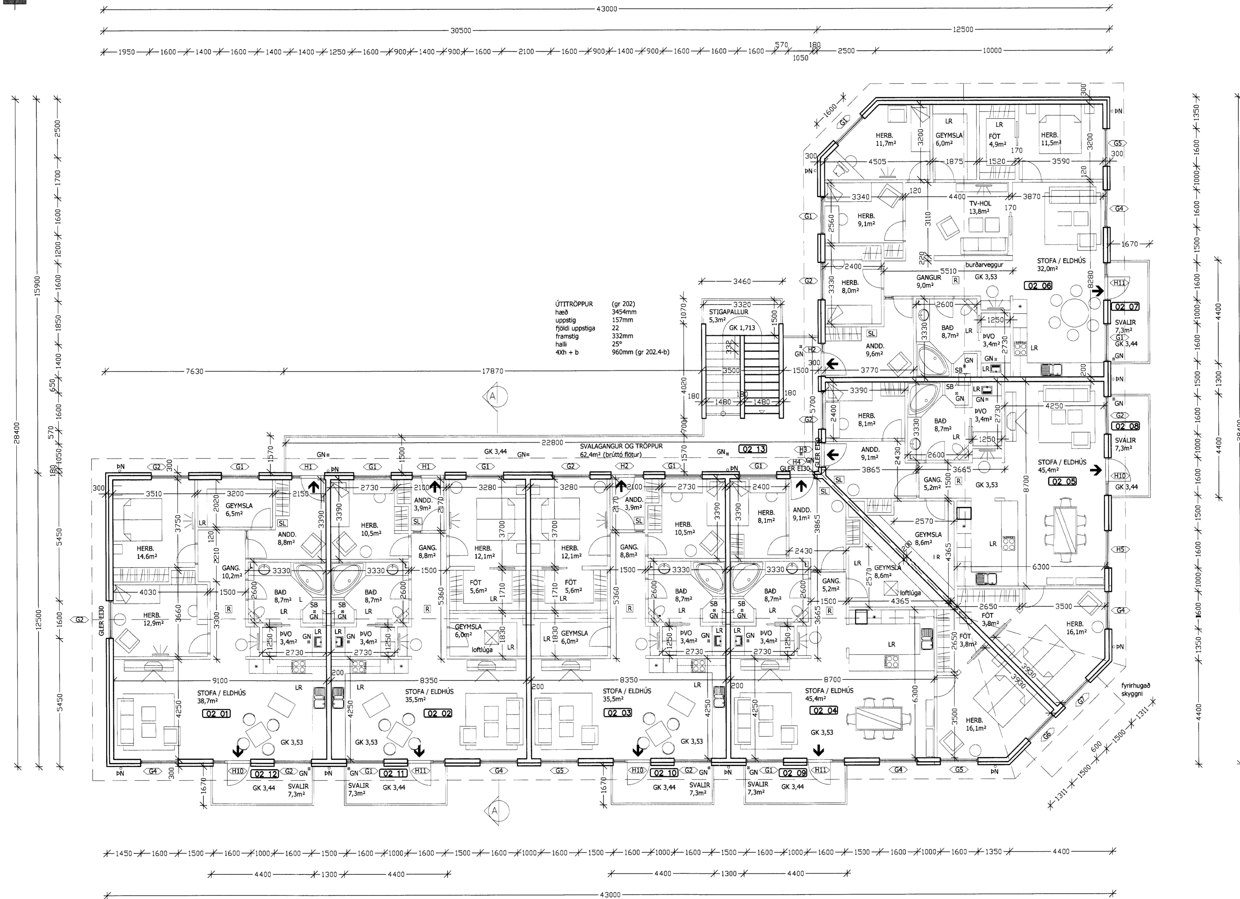
GRUNNMYND 2.HÆÐ 1:100
